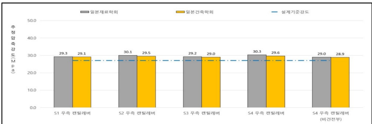
【그림 3.46】 상부구조 반발경도 시험결과(울산)
