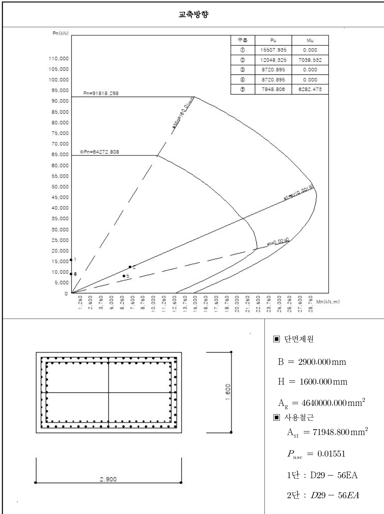
【그림 5.34】 교축방향 P-M상관도(P2)(부산)
