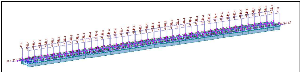
【그림 5.4】 합성전 고정하중(바닥판 하중) 재하도(부산)
