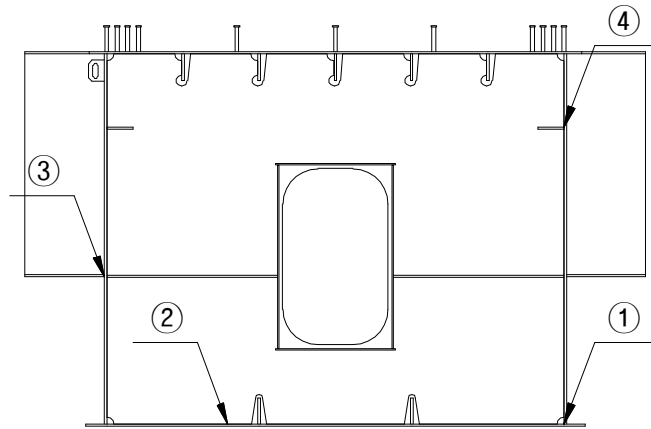
【표 5.22】 정모멘트부 검토위치 및 응력범주(부산)
