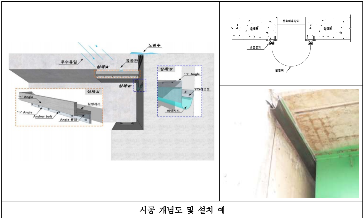
【그림 7.8】 유도배수시설 설치 모식도 및 설치 예
