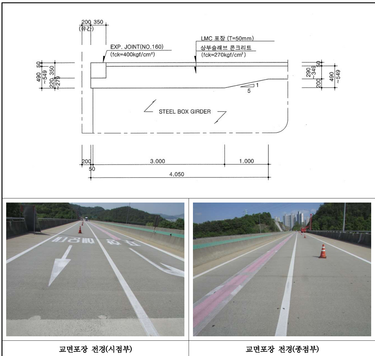
【사진 3.23】 교면포장 전경(부산)
