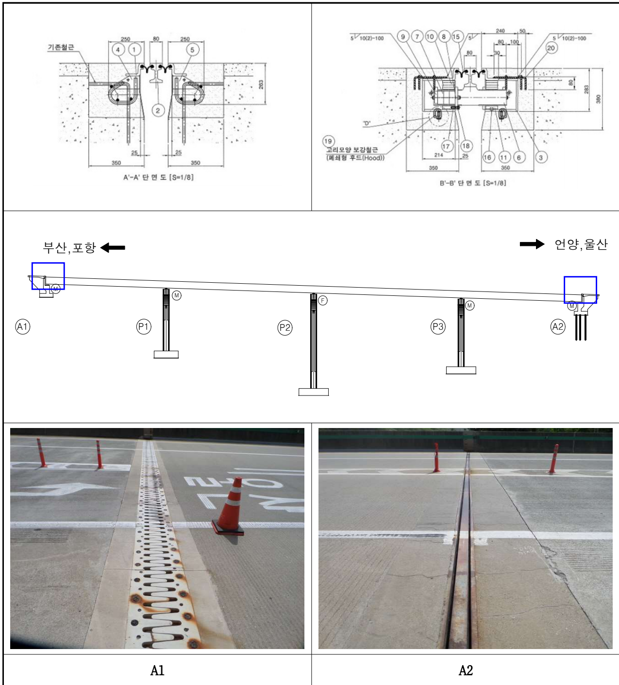
【그림 3.28】 신축이음장치 전경 및 상세도(울산)(계속)
