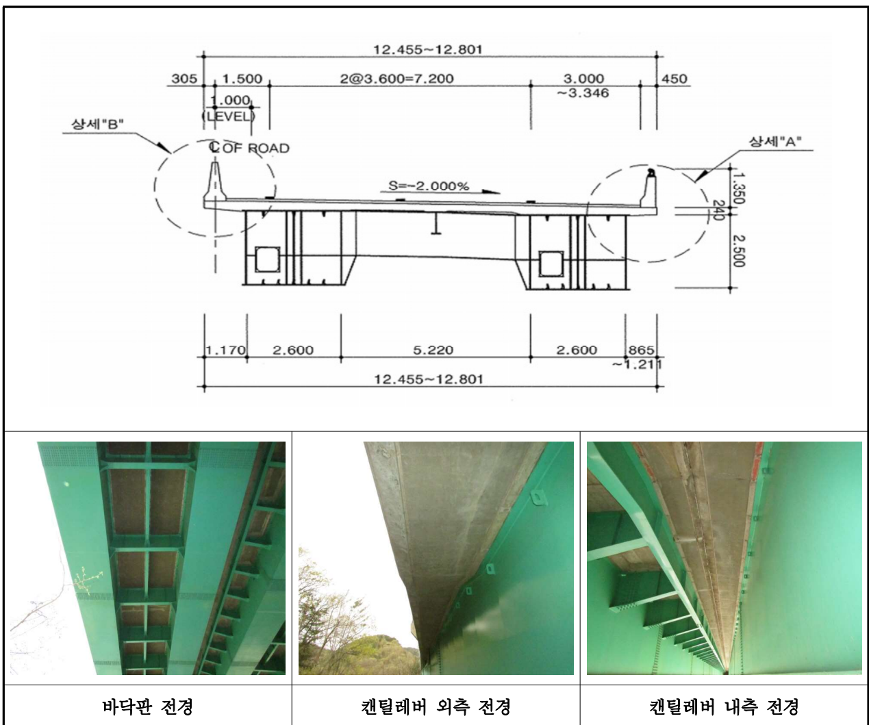
【사진 3.4】 바닥판 전경(부산)
