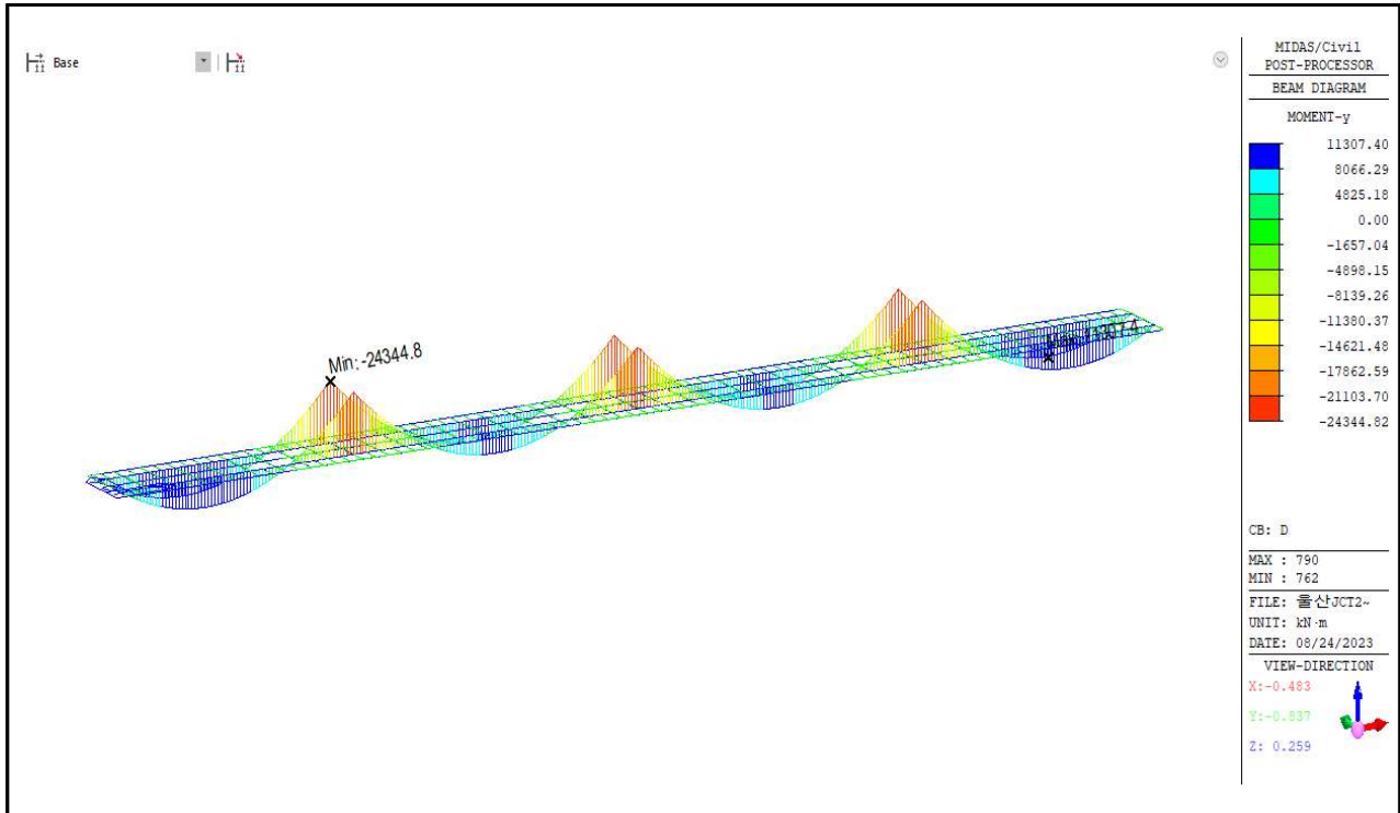
【그림 5.22】 합성전 고정하중에 의한 휨모멘트도(울산)
