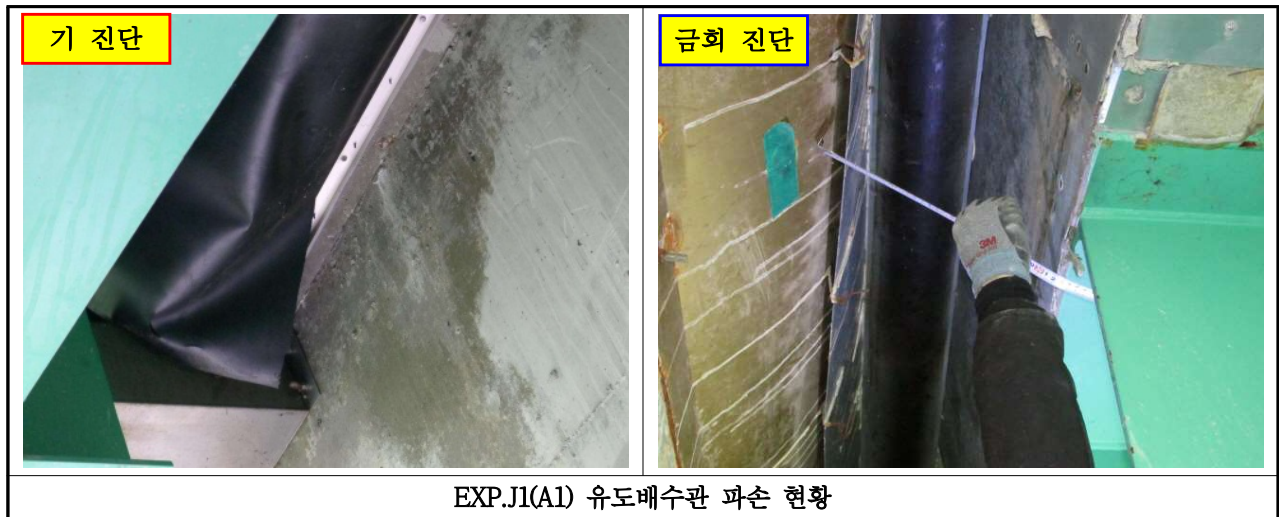
【표 3.90】신축이음장치 기 진단 결과와의 비교(울산)
