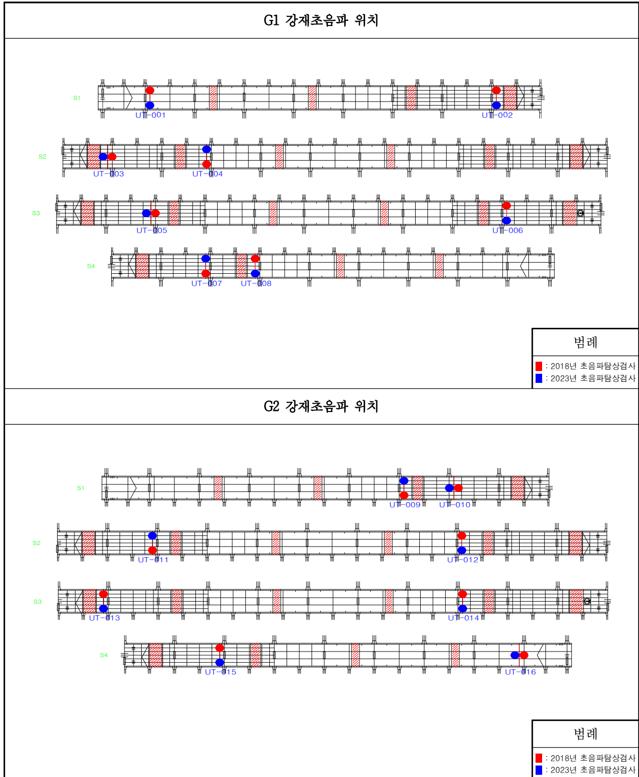
【그림 3.58】 강재 초음파 탐상시험(U.T) 위치도(울산)
