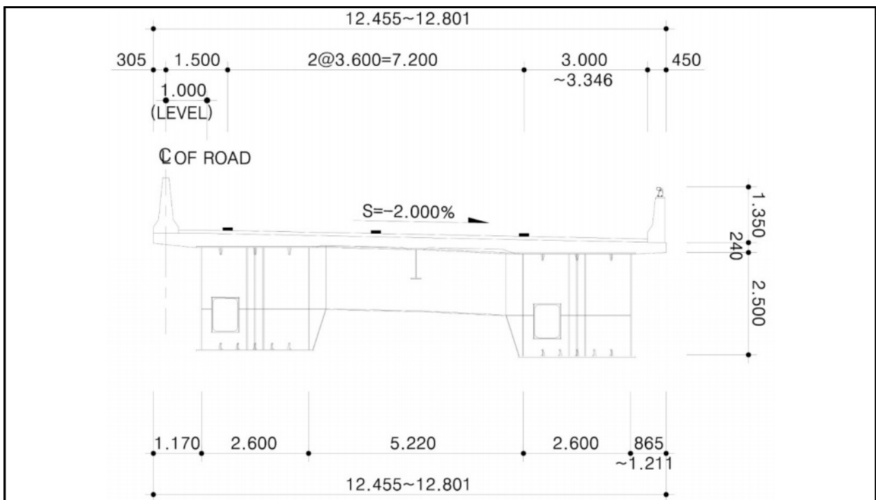
【그림 5.2】 횡단면도(부산)
