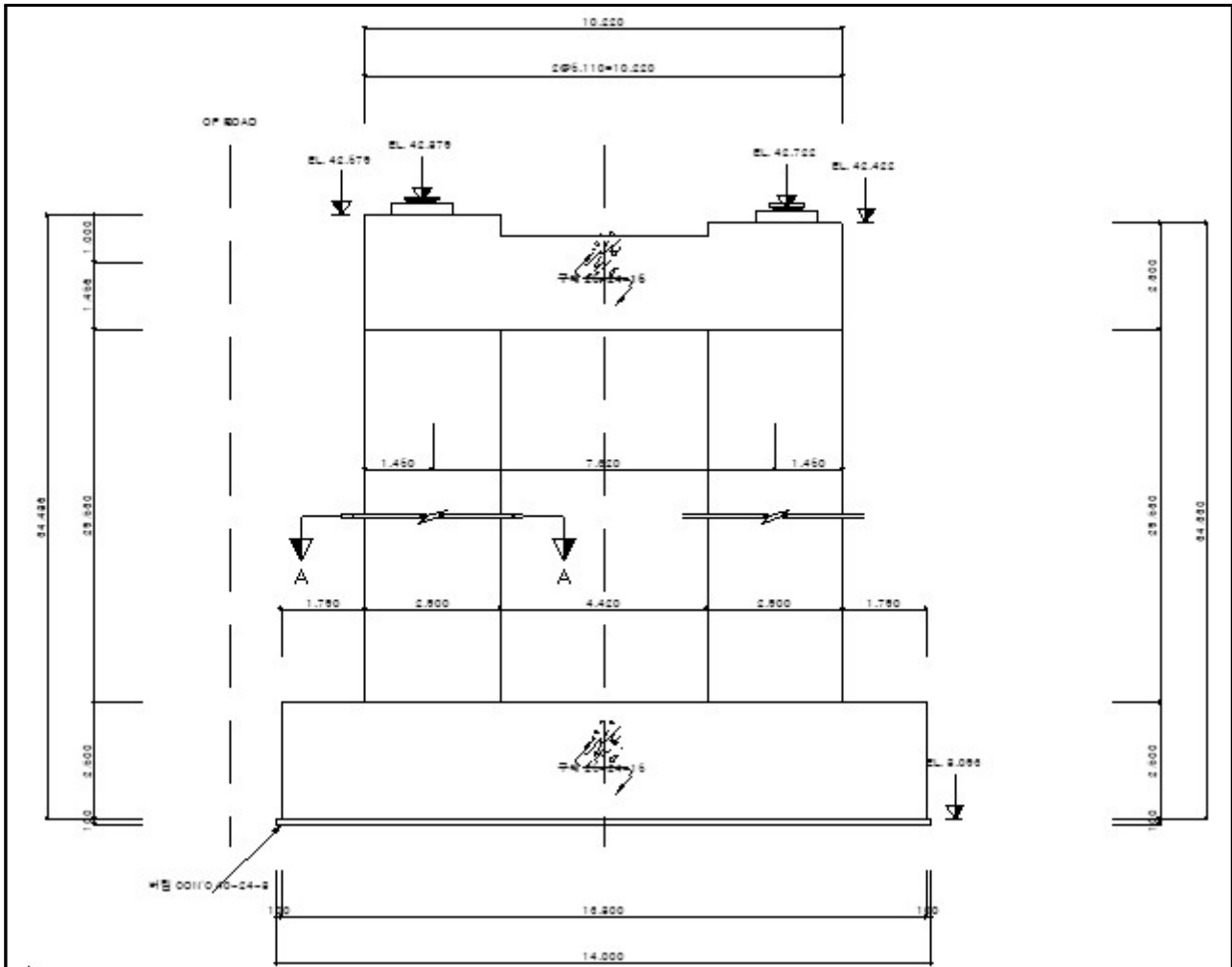
【그림 5.40】 해석단면(P2)(울산)
