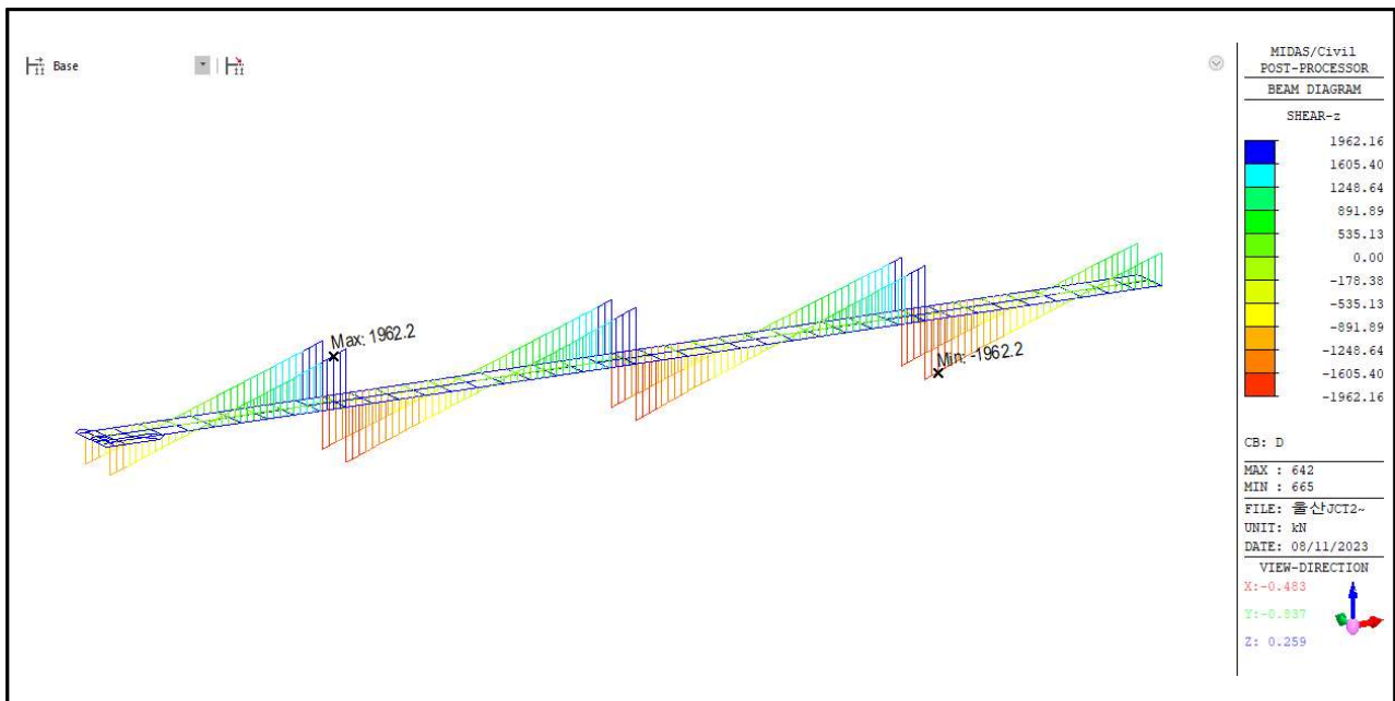
【그림 5.9】 합성전 고정하중에 의한 전단력도(부산)
