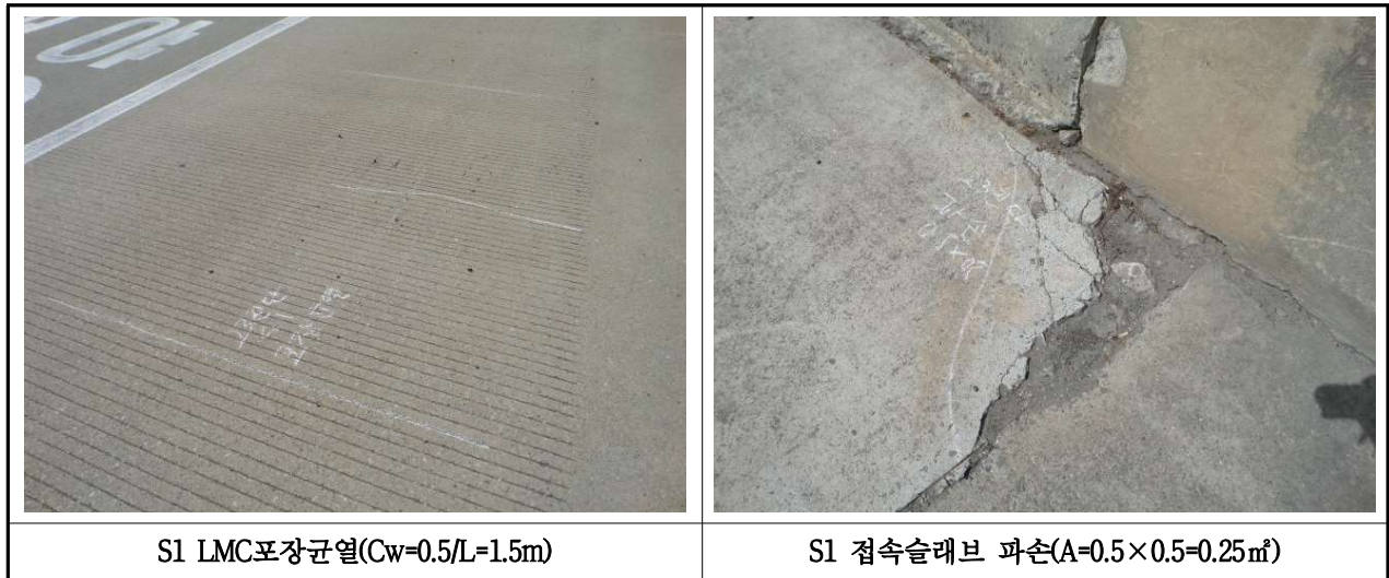
【사진 3.47】 교면포장 손상현황(울산)
