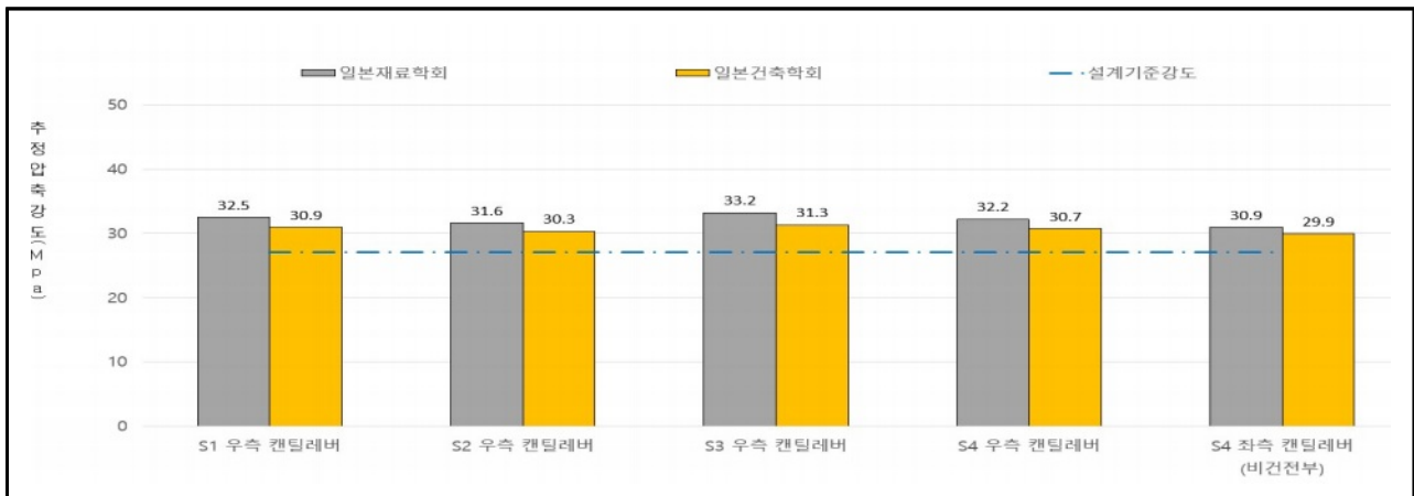
【그림 3.35】 상부구조 반발경도 시험결과(부산)
