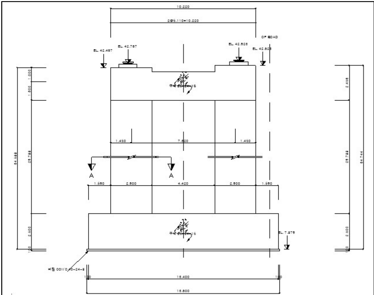
【그림 5.31】 해석단면(P2)(부산)
