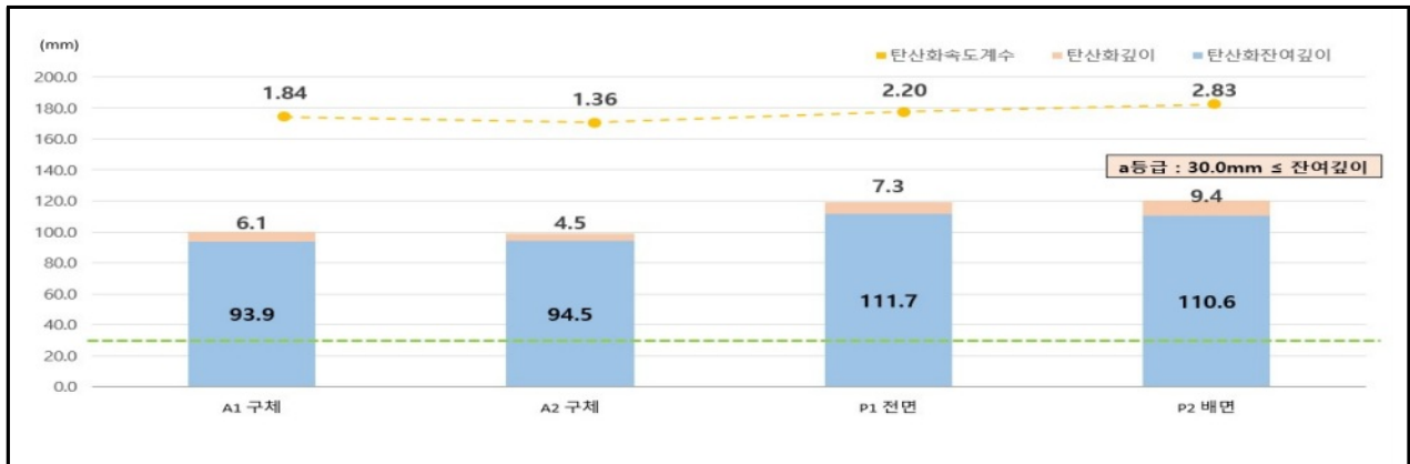
【그림 3.44】 하부구조 탄산화 깊이 측정 결과(부산)
