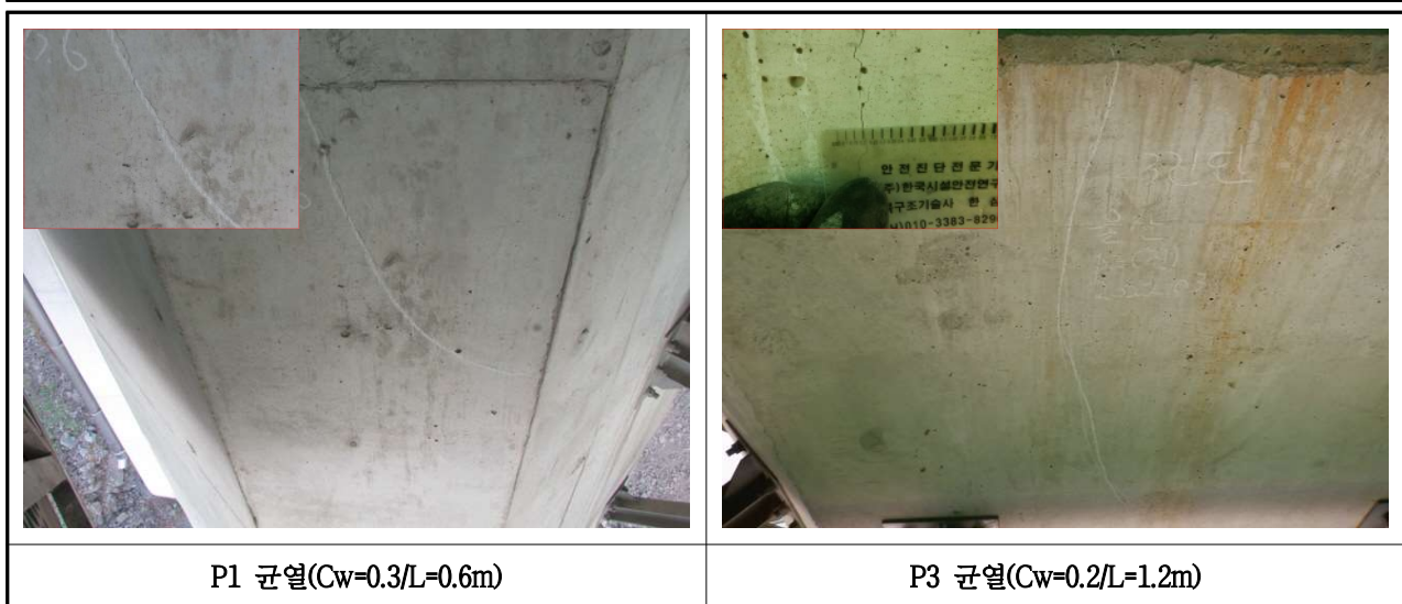
【사진 3.40】 교각 손상현황(울산)
