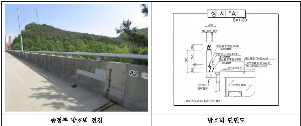
【사진 3.27】 난간 및 연석(방호벽) 전경 및 단면도(부산)(계속)
