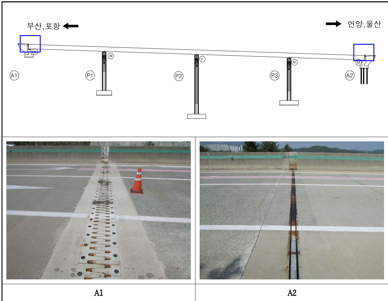
【그림 3.12】 신축이음장치 전경 및 배치도(부산)
