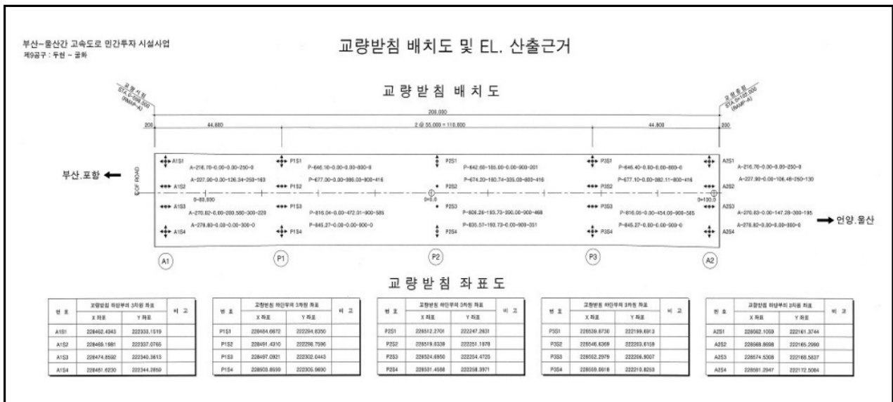
【그림 3.25】 교량받침 배치도(울산)
