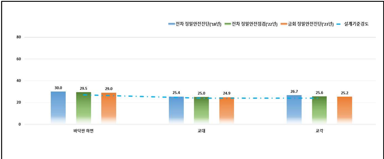
【그림 3.48】 전차 정밀안전진단 및 전차 정밀안전점검 결과 비교(울산)
