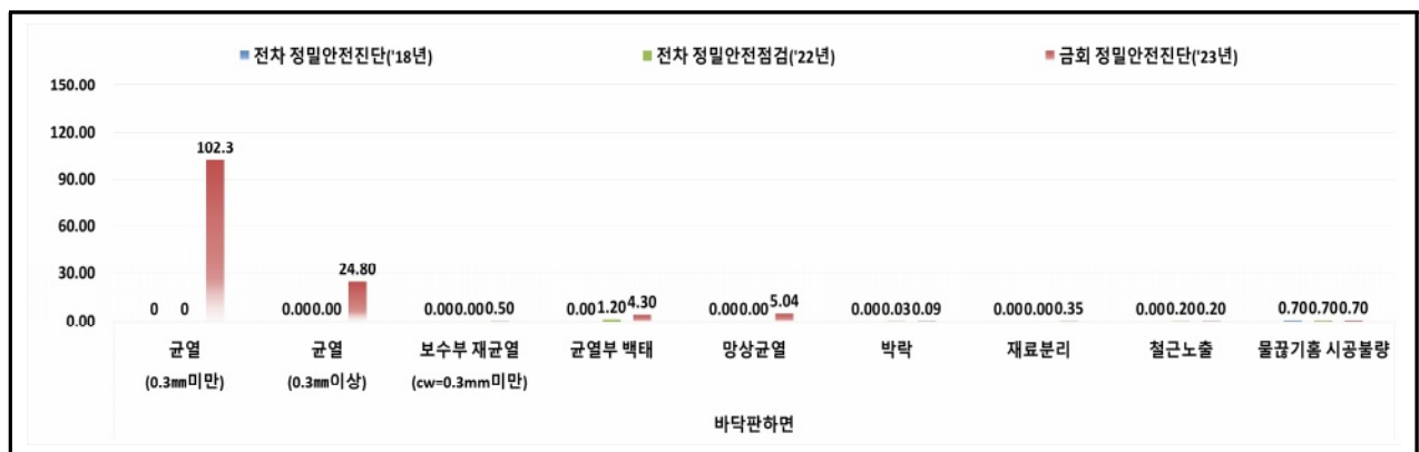
【그림 3.17】바닥판 하면 기 진단 결과와의 비교(울산)
