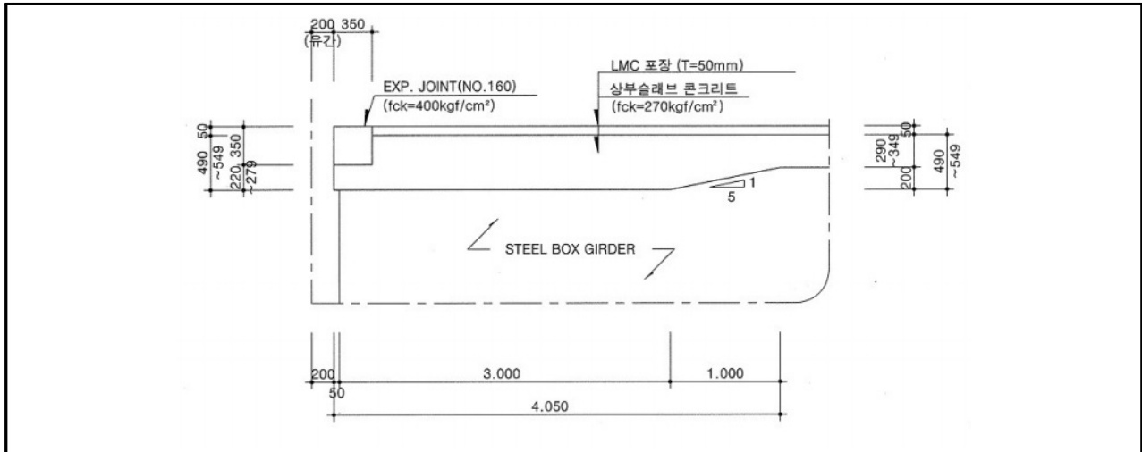
【그림 3.30】 교면포장 일반도(울산)
