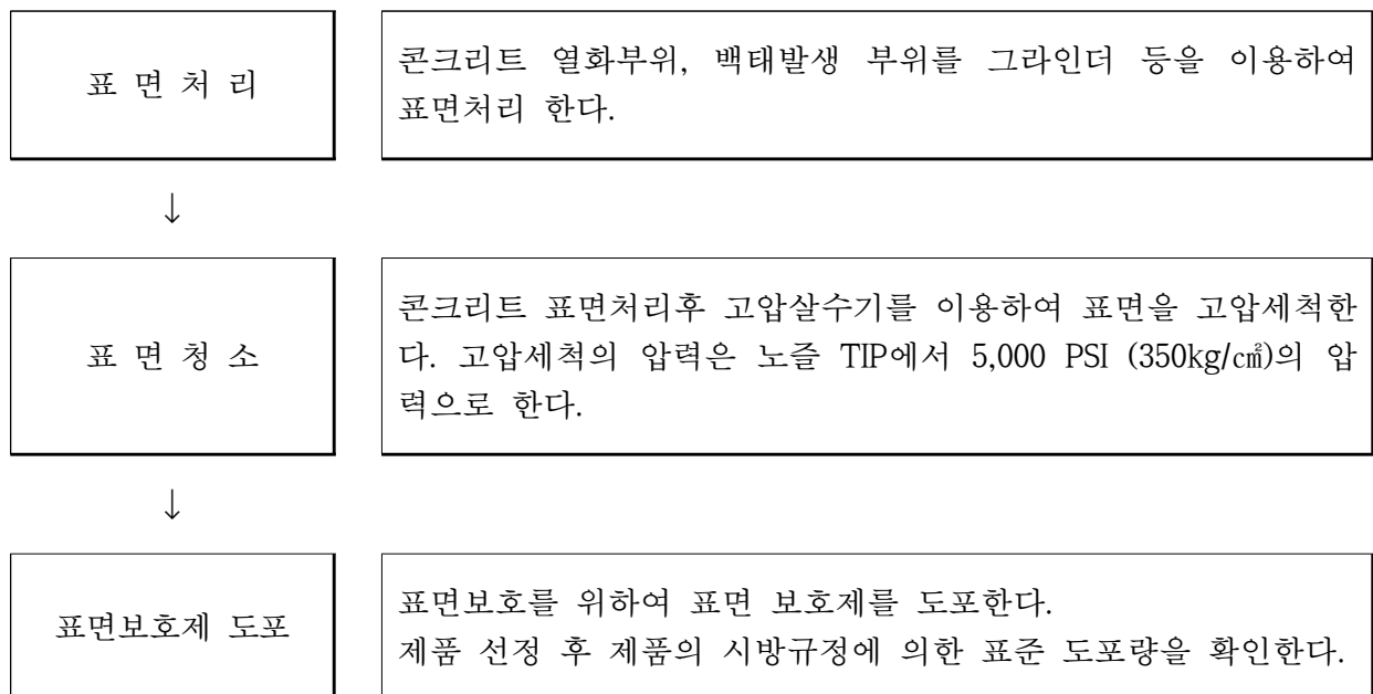
【그림 7.3】 콘크리트 표면처리 시공순서도
