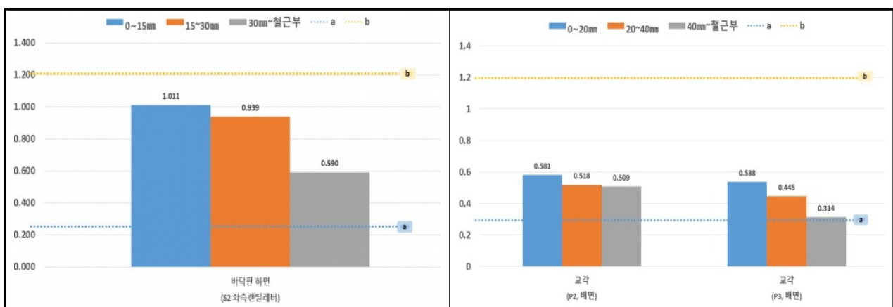
【그림 3.56】 염화물함유량 시험 결과(울산)
