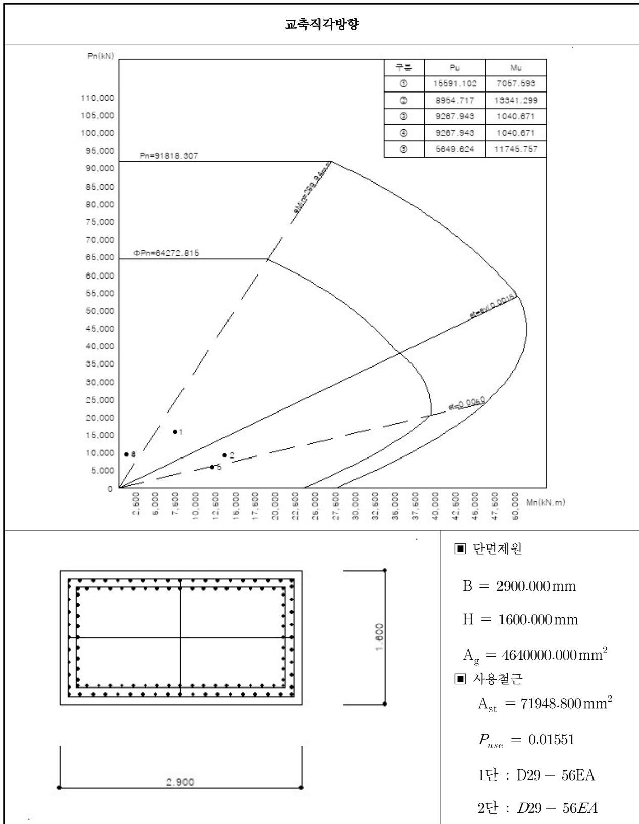
【그림 5.33】 교축직각방향 P-M상관도(P2)(부산)
