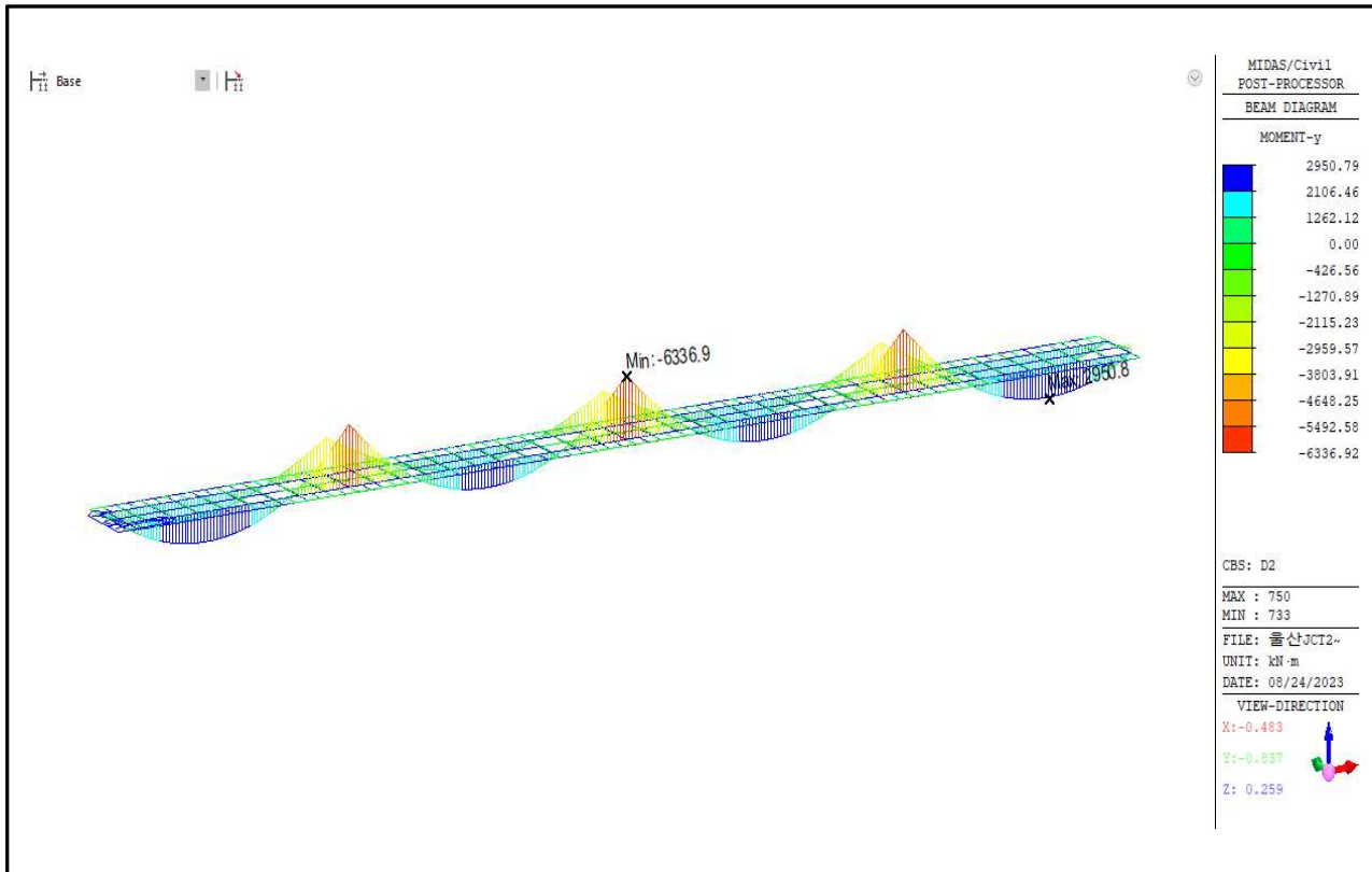
【그림 5.24】 합성후 고정하중에 의한 휨모멘트도(울산)
