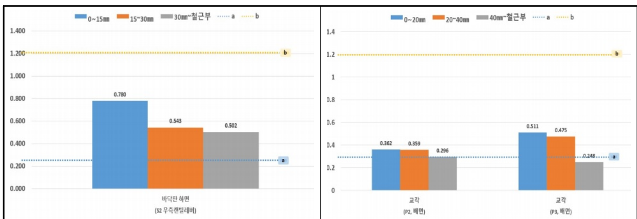
【그림 3.45】 염화물함유량 시험 결과(부산)
