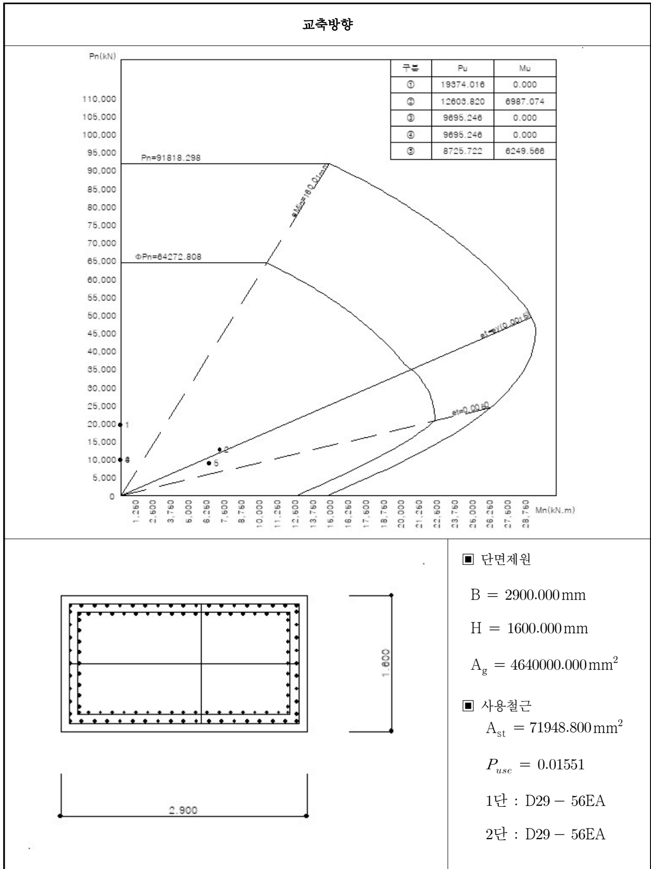
【그림 5.43】 교축방향 P-M상관도(P2)(울산)
