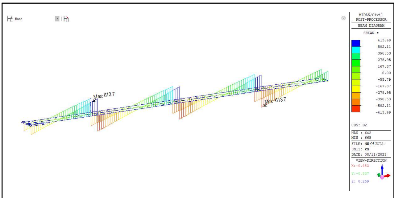
【그림 5.11】 합성후 고정하중에 의한 전단력도(부산)
