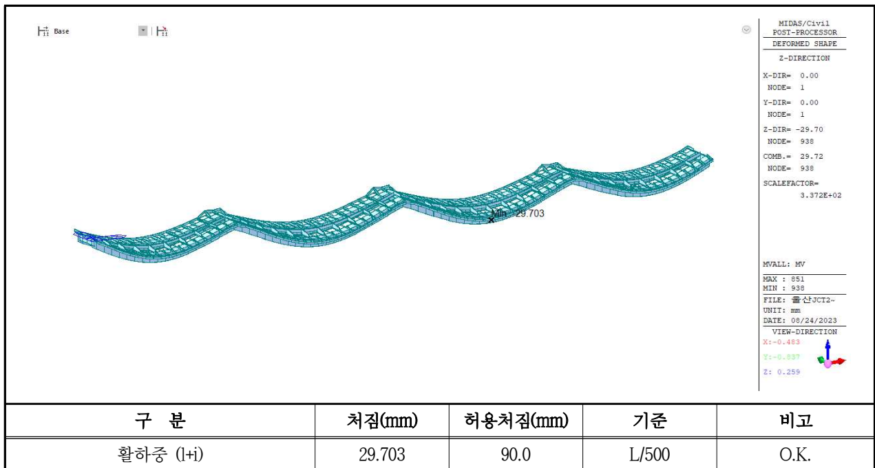
【그림 5.28】 처짐검토 결과(울산)
