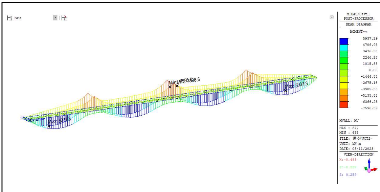
【그림 5.12】 활하중에 의한 휨모멘트도(부산)
