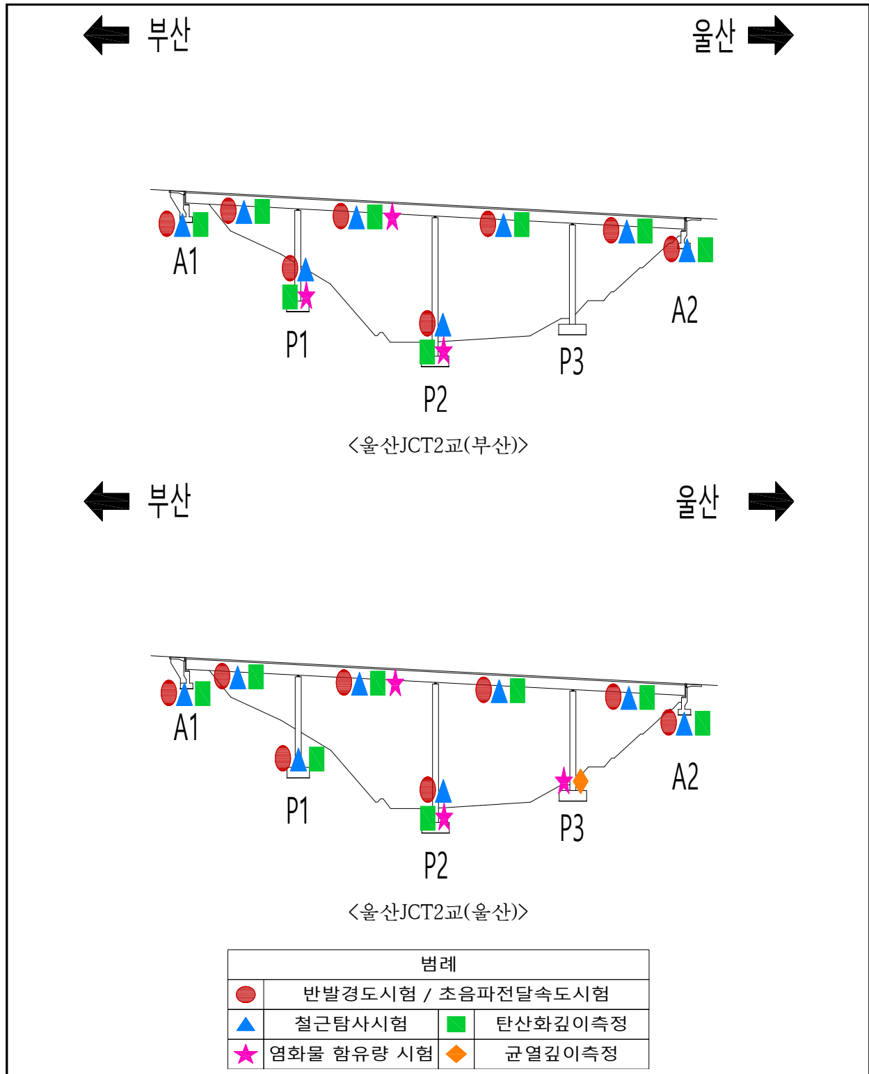
【그림 3.34】 콘크리트 내구성조사 위치도
