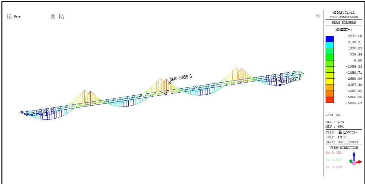
【그림 5.10】 합성후 고정하중에 의한 휨모멘트도(부산)
