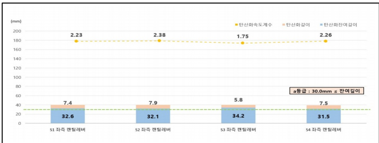
【그림 3.54】 상부구조 탄산화 깊이 측정 결과(울산)
