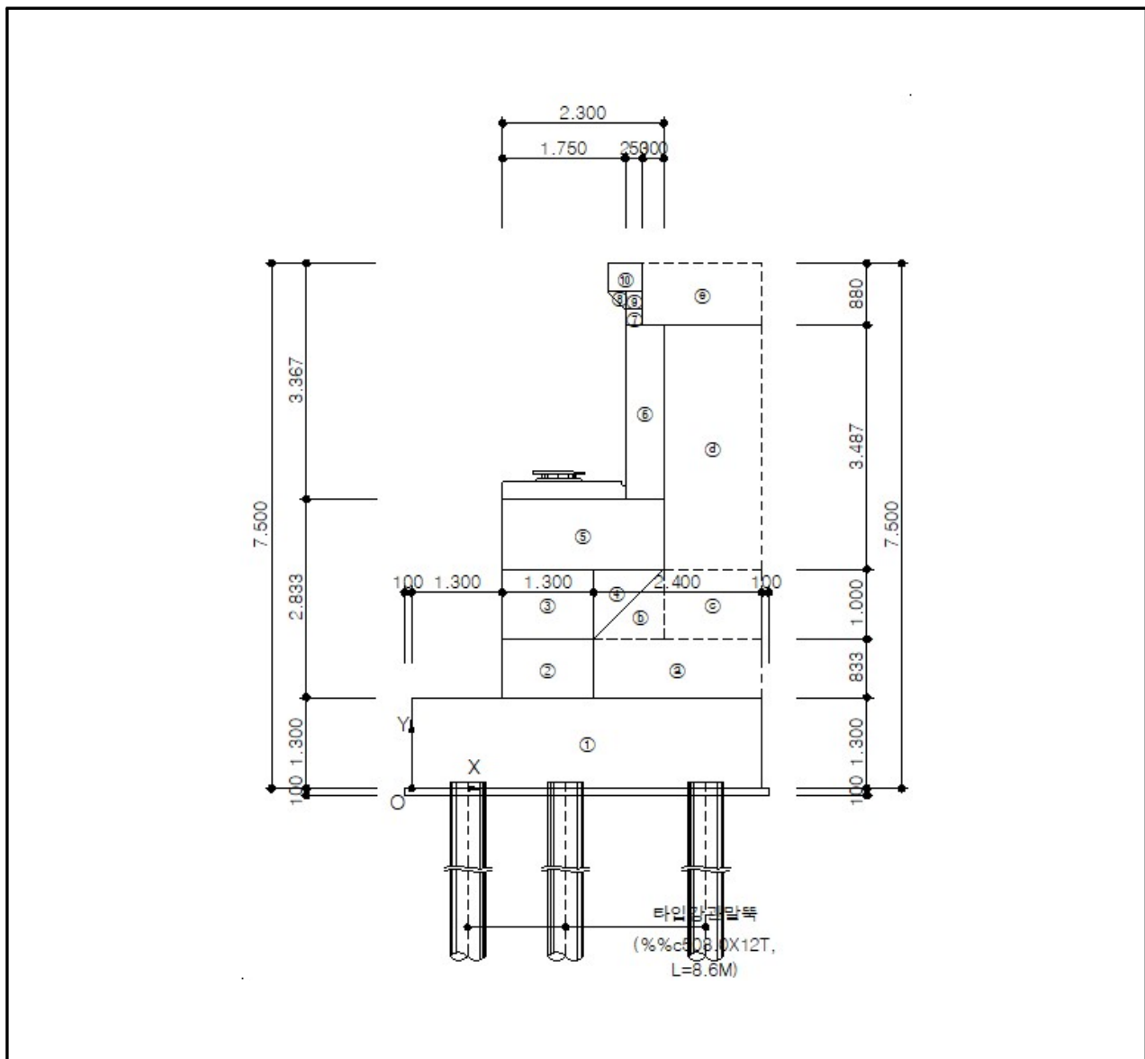
【그림 5.39】 해석단면(A2)(울산)
