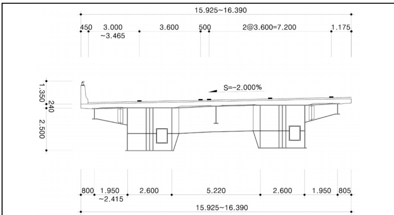
【그림 5.16】 횡단면도(울산)
