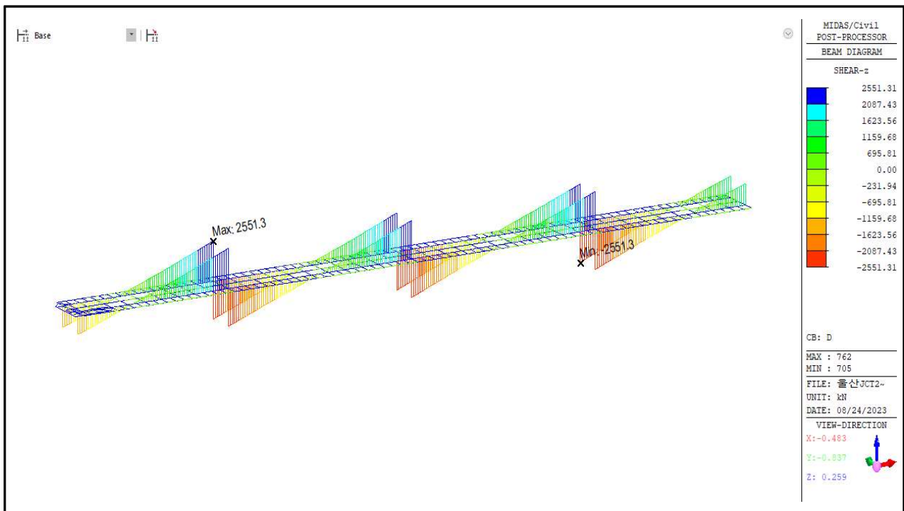
【그림 5.23】 합성전 고정하중에 의한 전단력도(울산)
