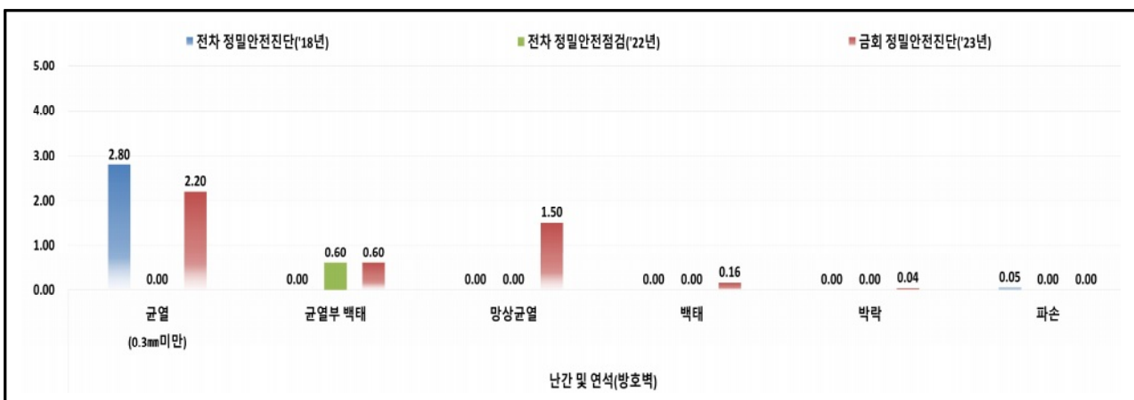
【그림 3.33】 난간 및 연석(방호벽) 기 진단 결과와의 비교(울산)
