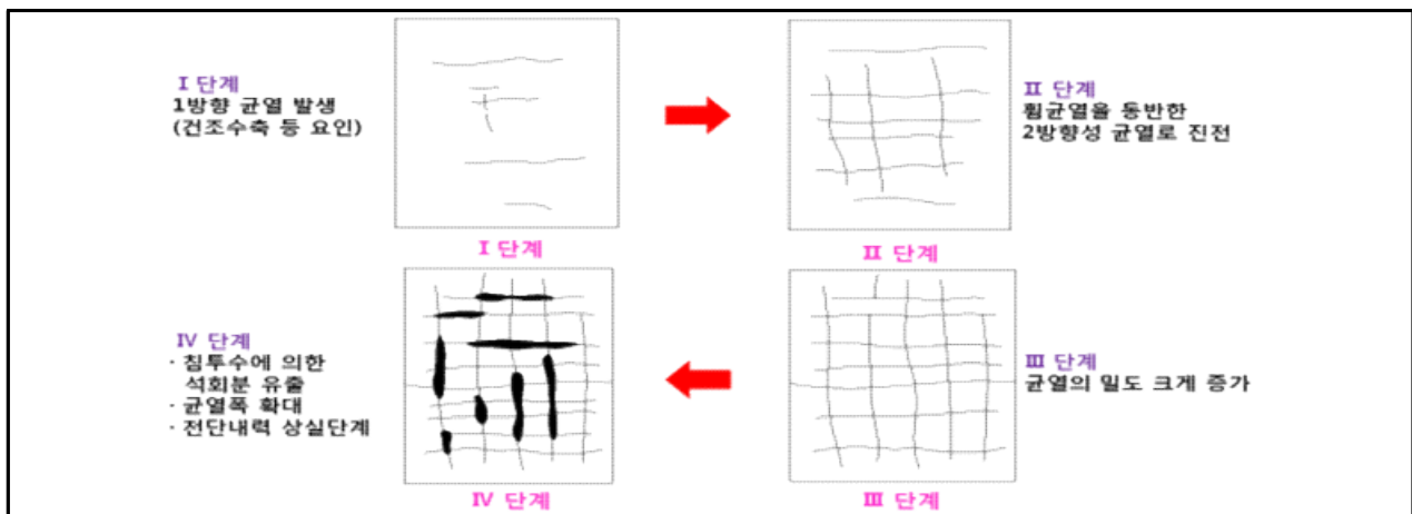
【그림 3.2】 콘크리트 바닥판의 균열진전 개요도(부산)
