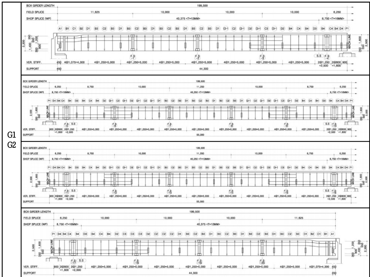
【그림 5.17】 단면배치도(울산)
