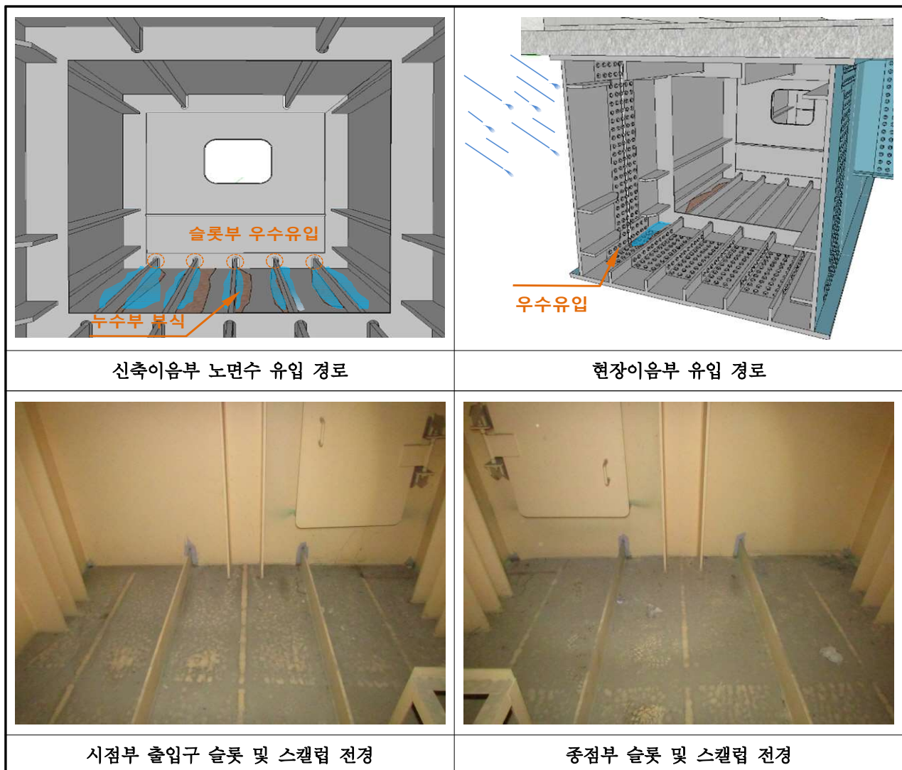
【사진 3.9】 강박스 거더 내부 우수 유입경로(부산)
