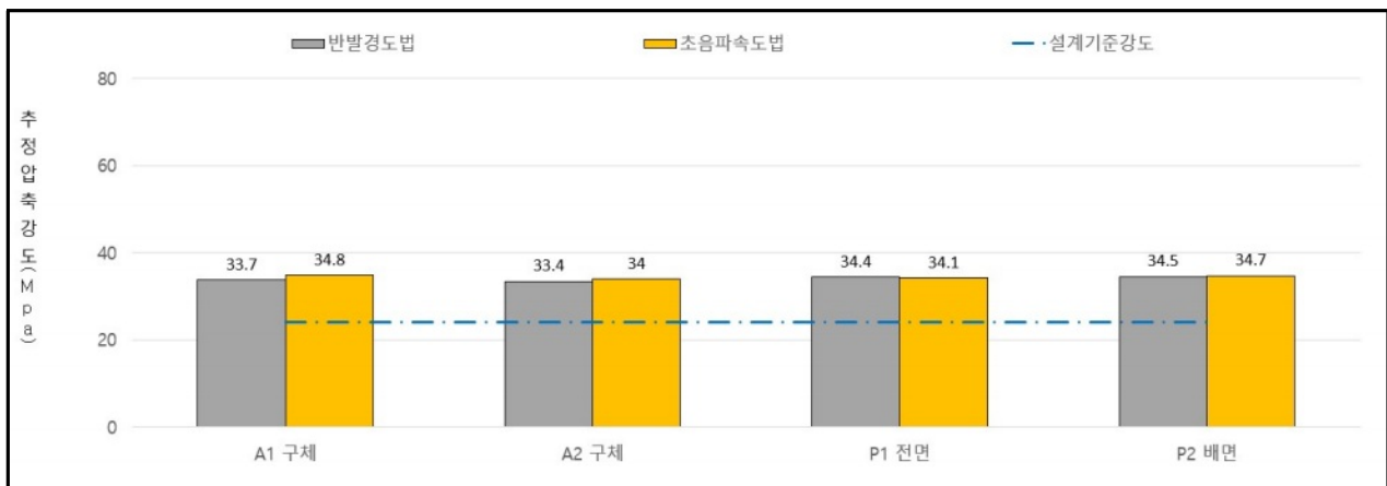
【그림 3.41】하부구조 추정비파괴강도 결과 그래프(부산)
