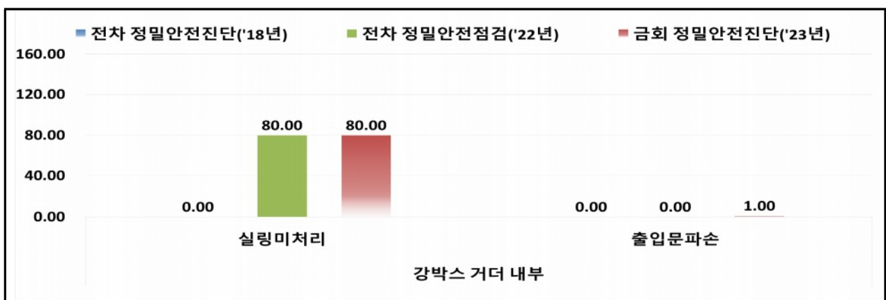
【그림 3.20】거더 내부 기 진단 결과와의 비교(울산)
