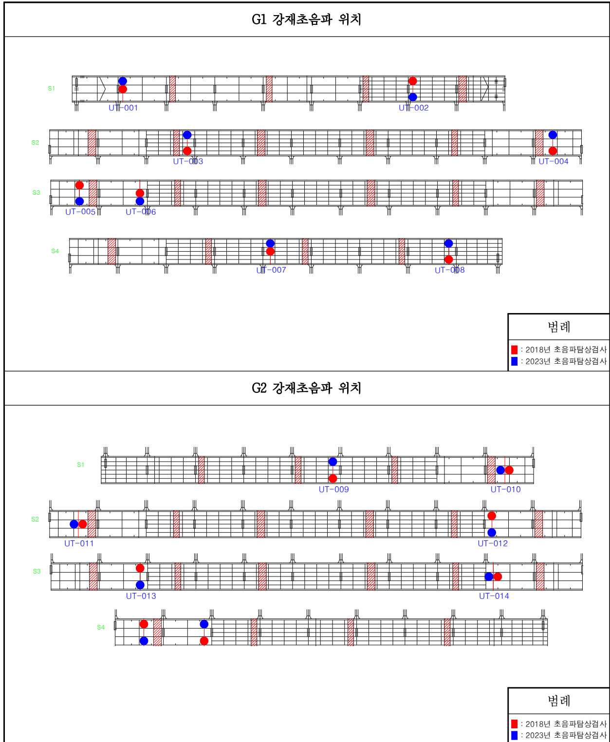
【그림 3.57】 강재 초음파 탐상시험(U.T) 위치도(부산)
