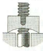
<Spring nut>
