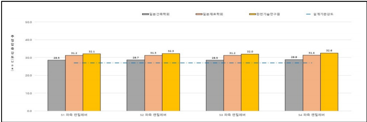
【그림 3.49】 상부구조 초음파 전달속도 시험결과(울산)
