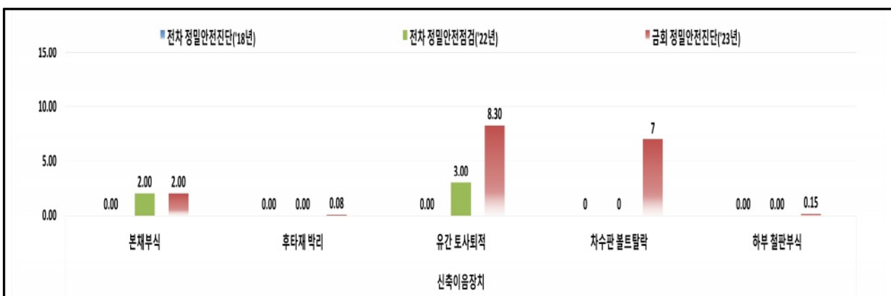
【그림 3.13】 신축이음장치 기 진단 결과와의 비교(부산)
