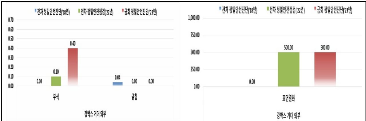
【그림 3.5】 강박스 거더 외부 기 진단 결과와의 비교(부산)
