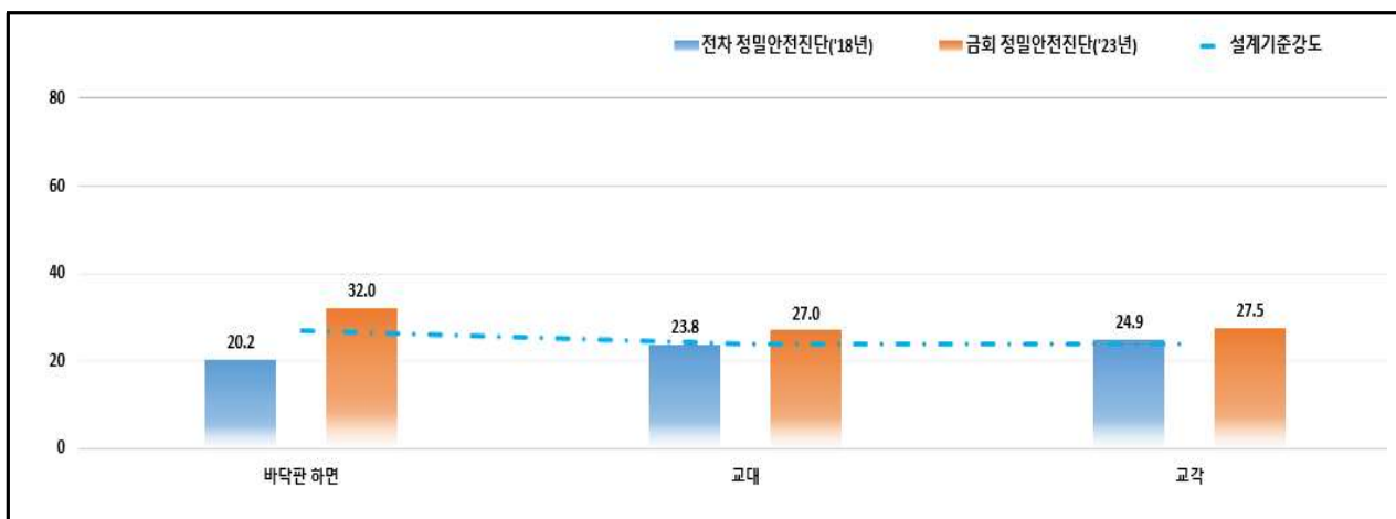
【그림 3.51】 전차 정밀안전진단 결과 비교(울산)
