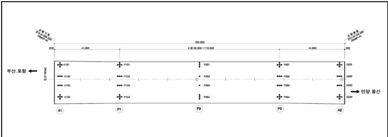
【그림 5.29】 받침배치도(울산)
