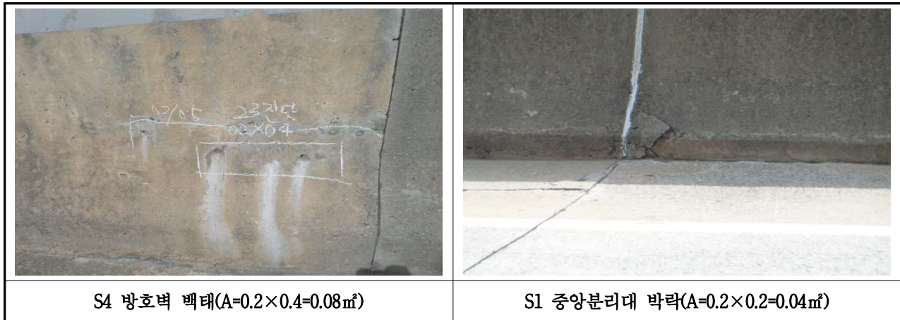
【사진 3.51】 난간 및 연석(방호벽) 손상현황(울산)(계속)
