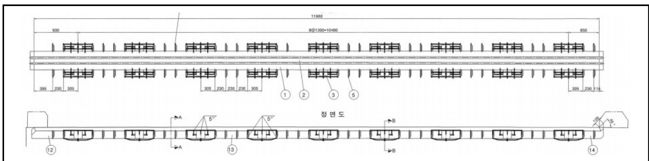
【그림 3.28】 신축이음장치 전경 및 상세도(울산)
