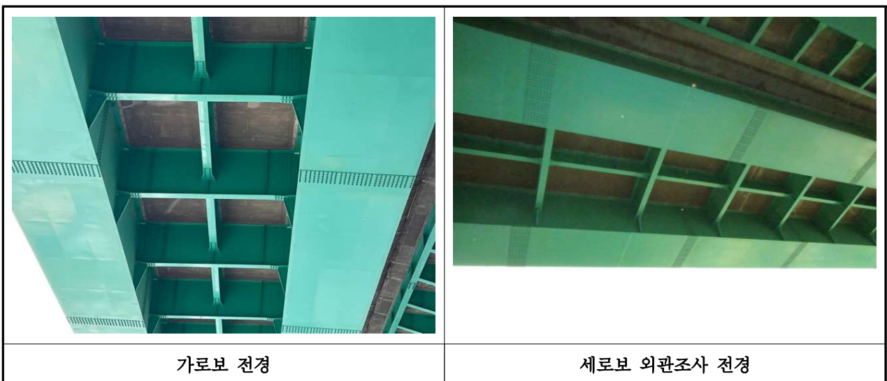
【사진 3.11】 2차부재(가로보, 세로보) 전경(부산)
