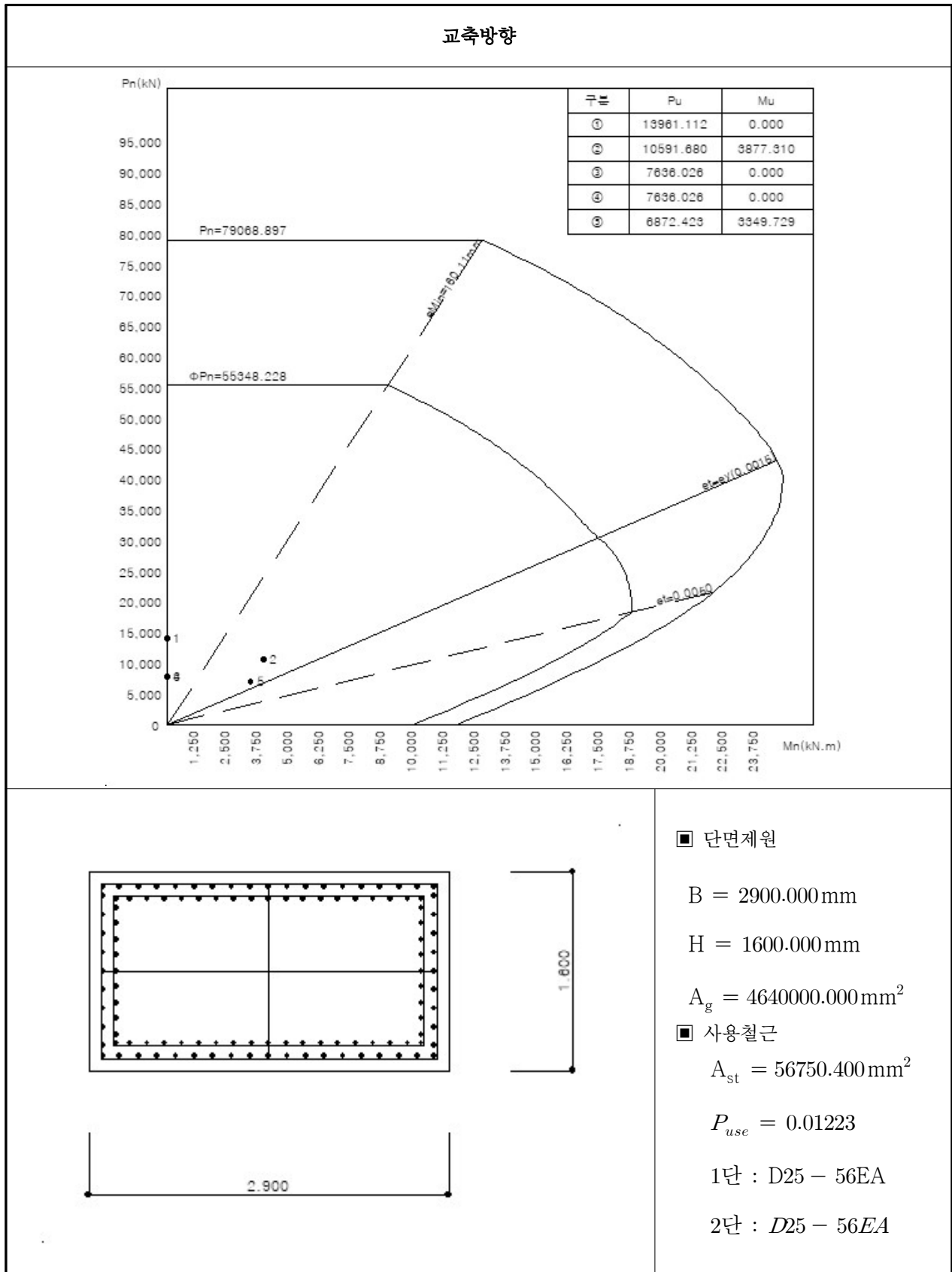
【그림 5.38】 교축방향 P-M상관도(P3)(부산)
