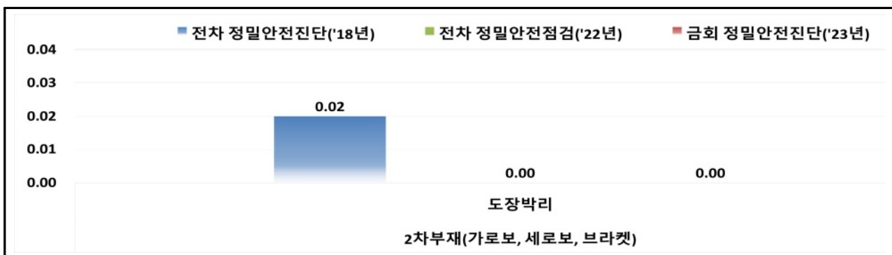
【그림 3.22】 2차부재(가로보, 세로보, 브라켓) 기 진단 결과와의 비교(울산)
