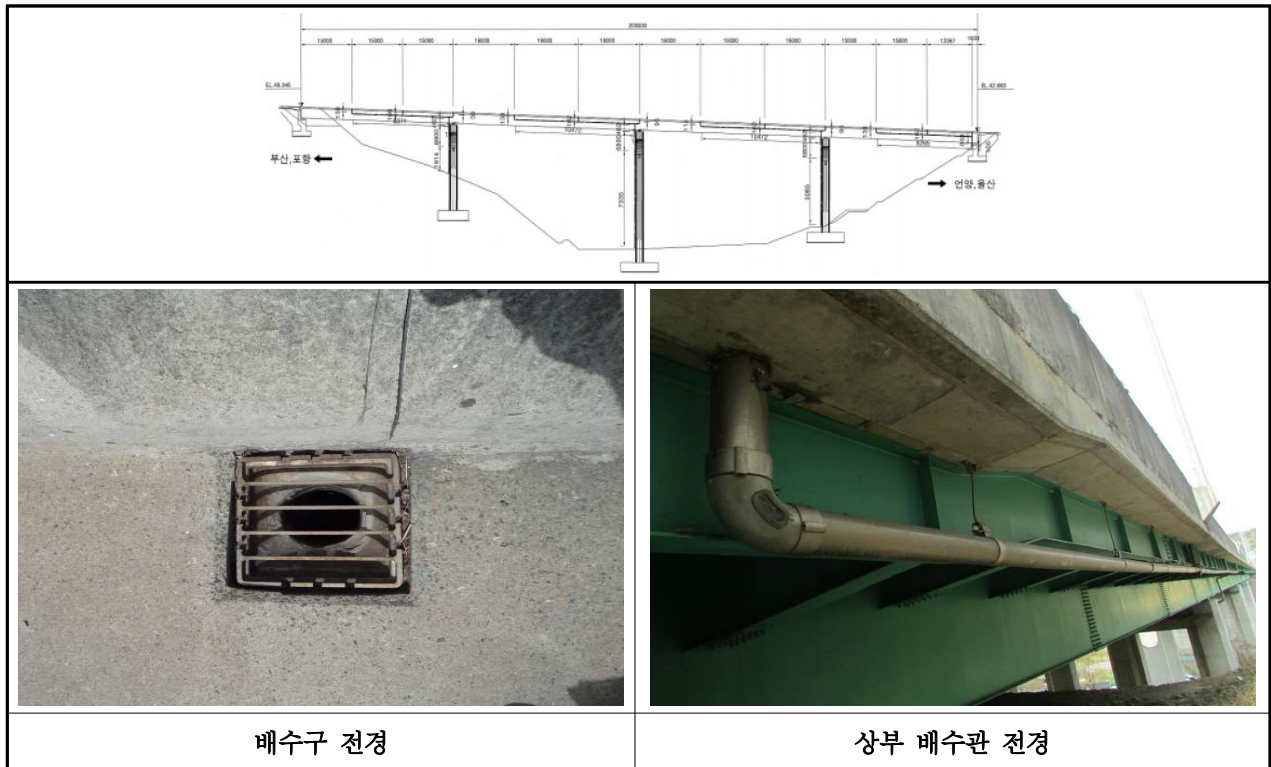
【사진 3.48】 배수시설 위치도 및 전경(울산)
