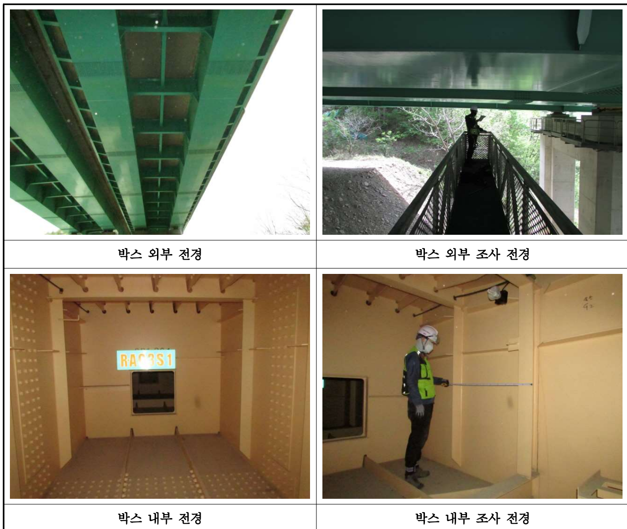
【사진 3.31】 강박스 거더 전경(울산)
