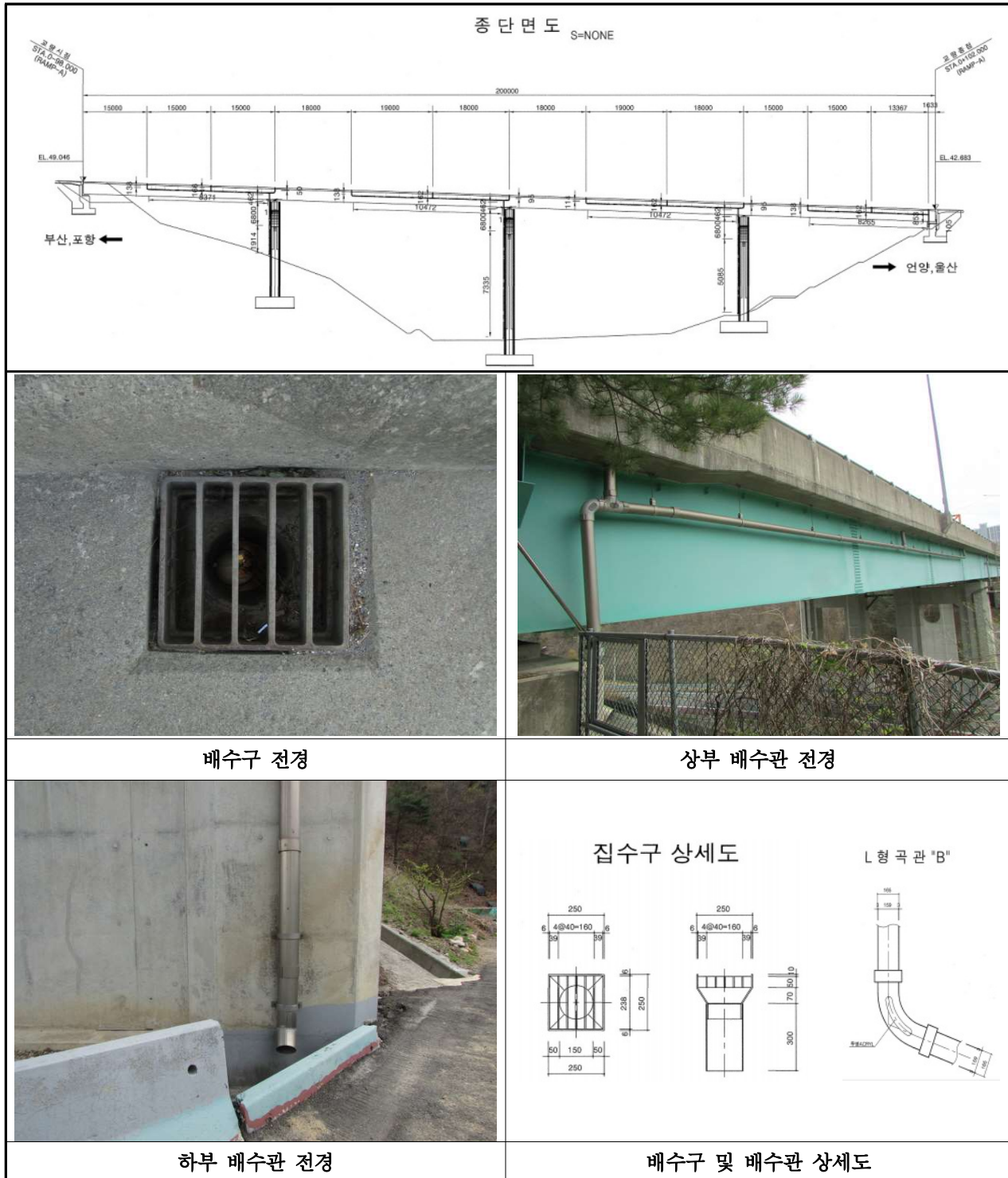
【사진 3.25】 배수시설 위치도 및 전경(부산)
