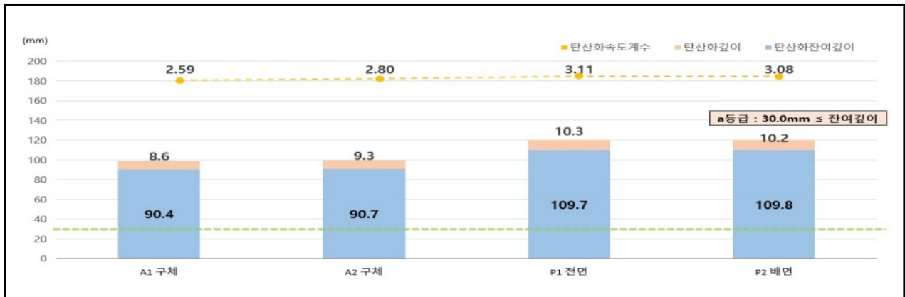
【그림 3.55】하부구조 탄산화 깊이 측정 결과(울산)
