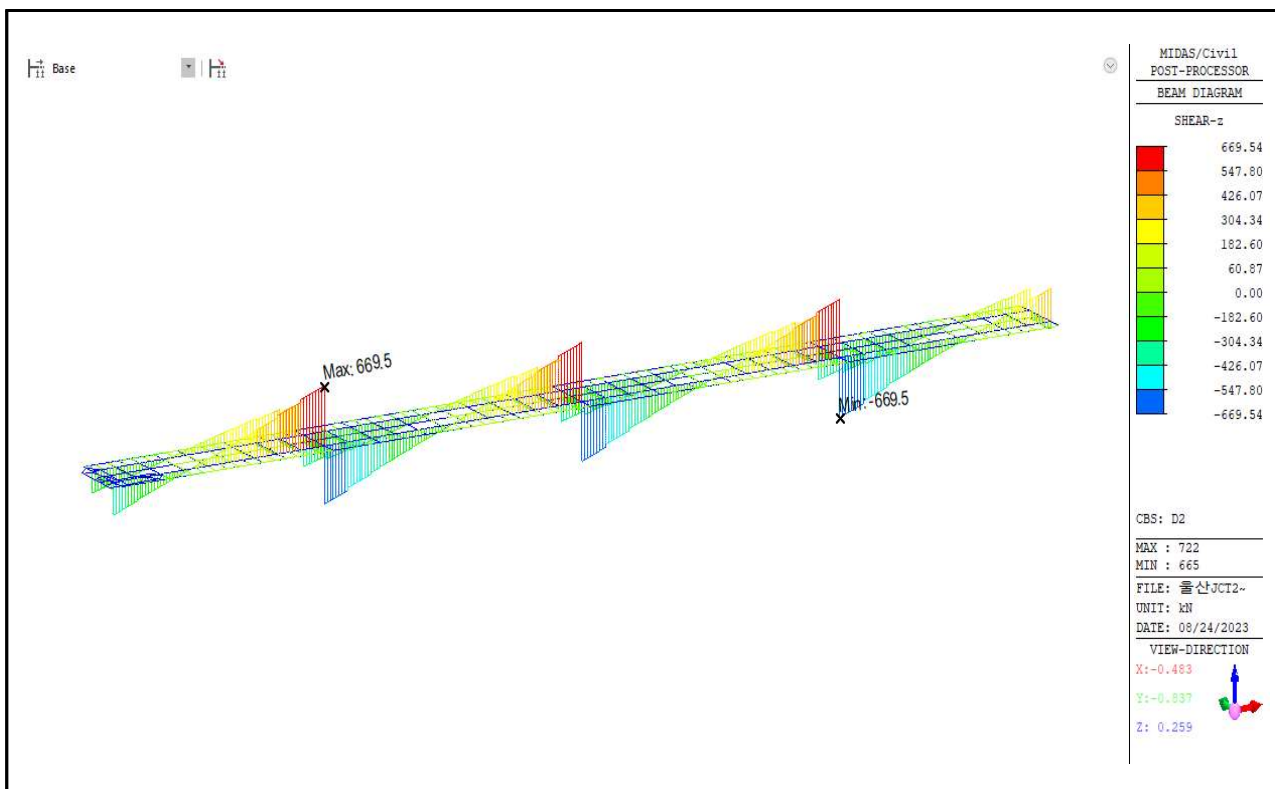
【그림 5.25】 합성후 고정하중에 의한 전단력(울산)
