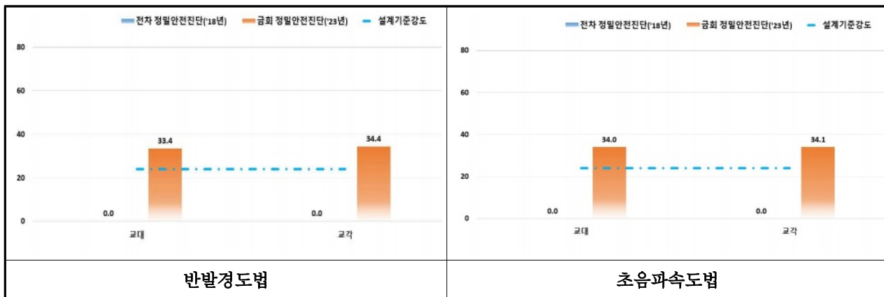
【그림 3.42】 전차 정밀안전진단 추정 비파괴 강도 결과와 비교(부산)
