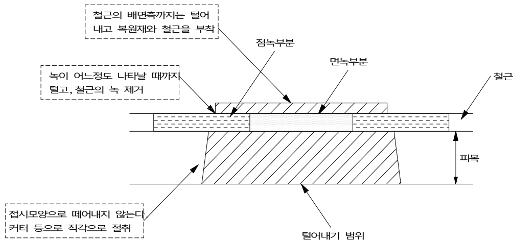
【그림 7.5】 단면복구(보수) 상세도
