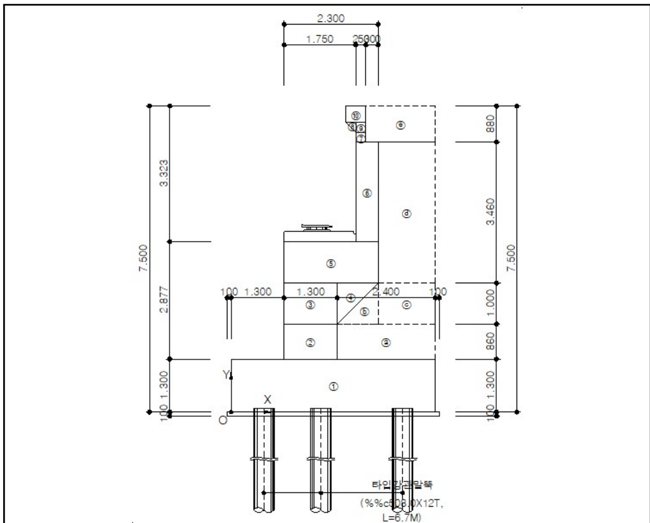
【그림 5.30】 해석단면(A2)(부산)
