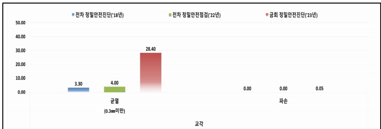
【그림 3.7】 교각 기 진단 결과와의 비교(부산)
