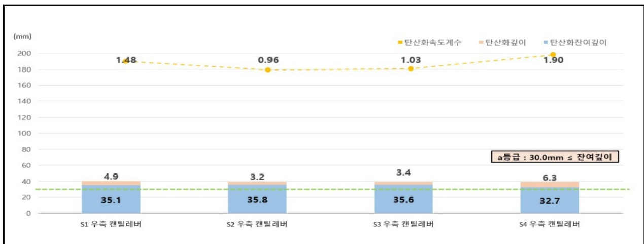
【그림 3.43】 상부구조 탄산화 깊이 측정 결과(부산)
