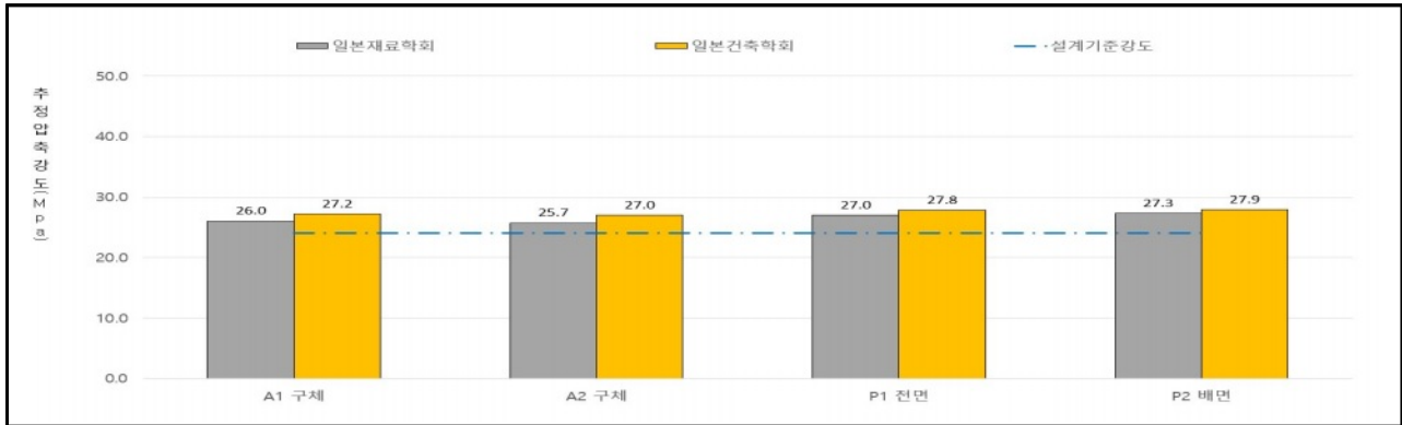
【그림 3.36】하부구조 반발경도 시험결과(부산)
