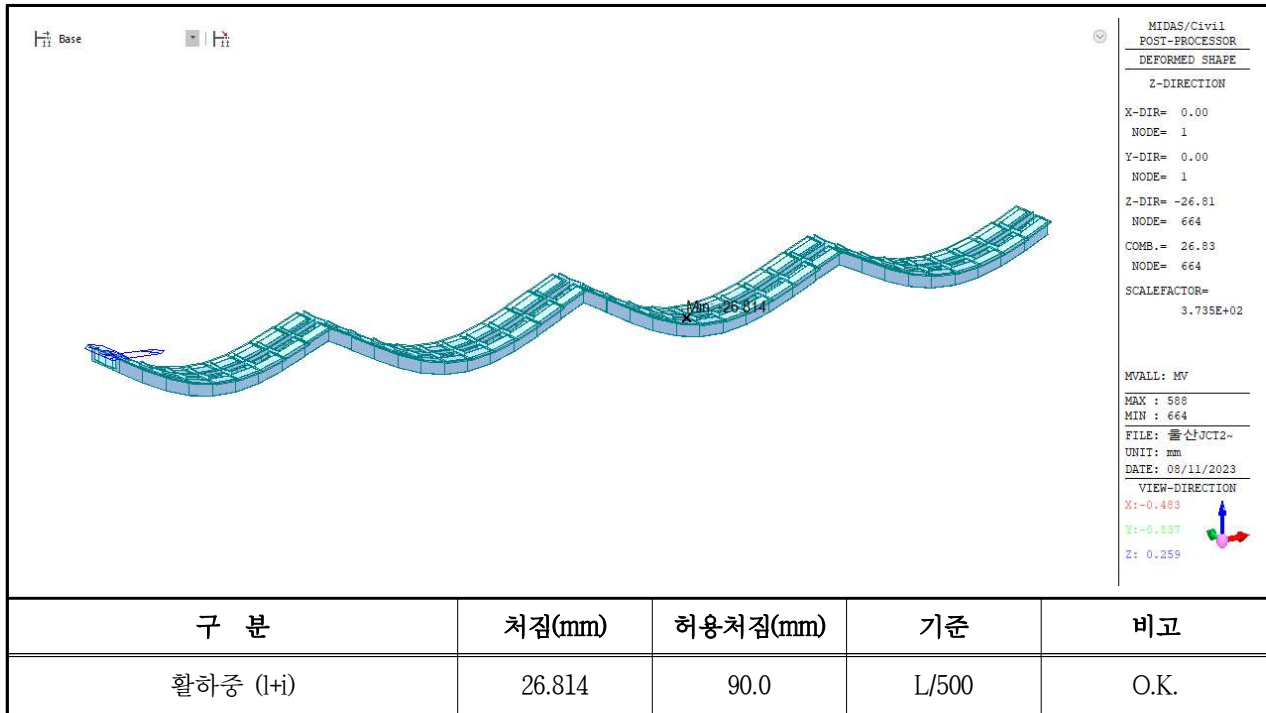
【그림 5.14】 처짐검토 결과(부산)
