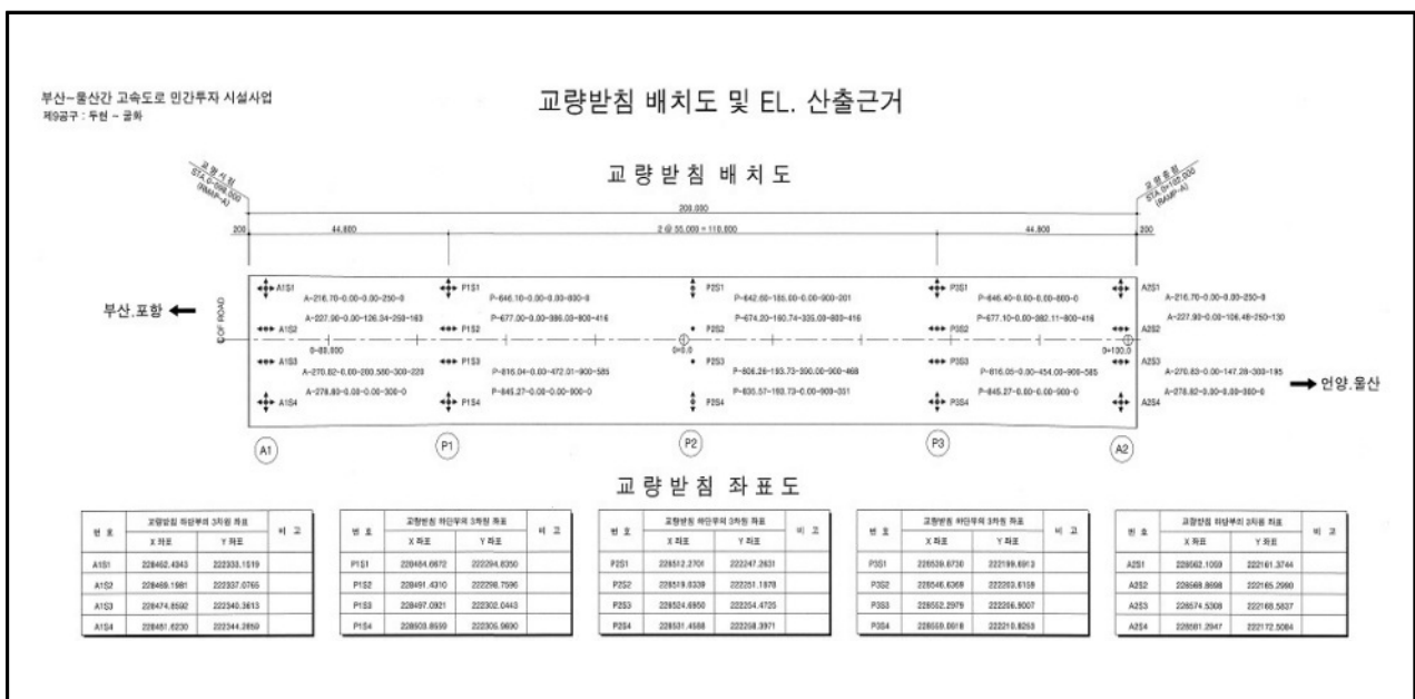
【그림 3.8】 교량받침 배치도(부산)
