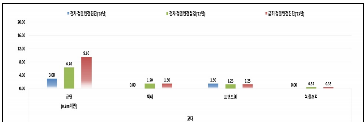
【그림 3.6】 교대 기 점검 결과와의 비교(부산)
