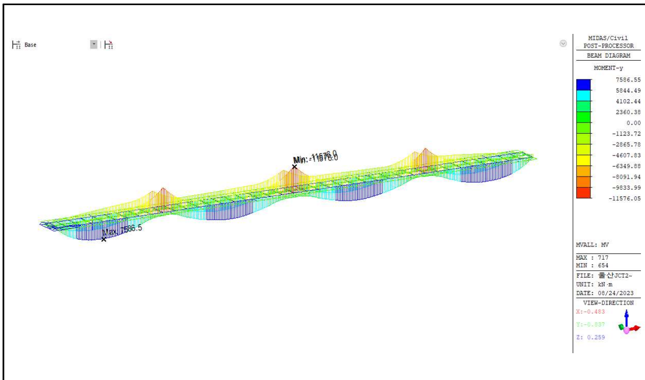
【그림 5.26】 활하중에 의한 휨모멘트도(울산)
