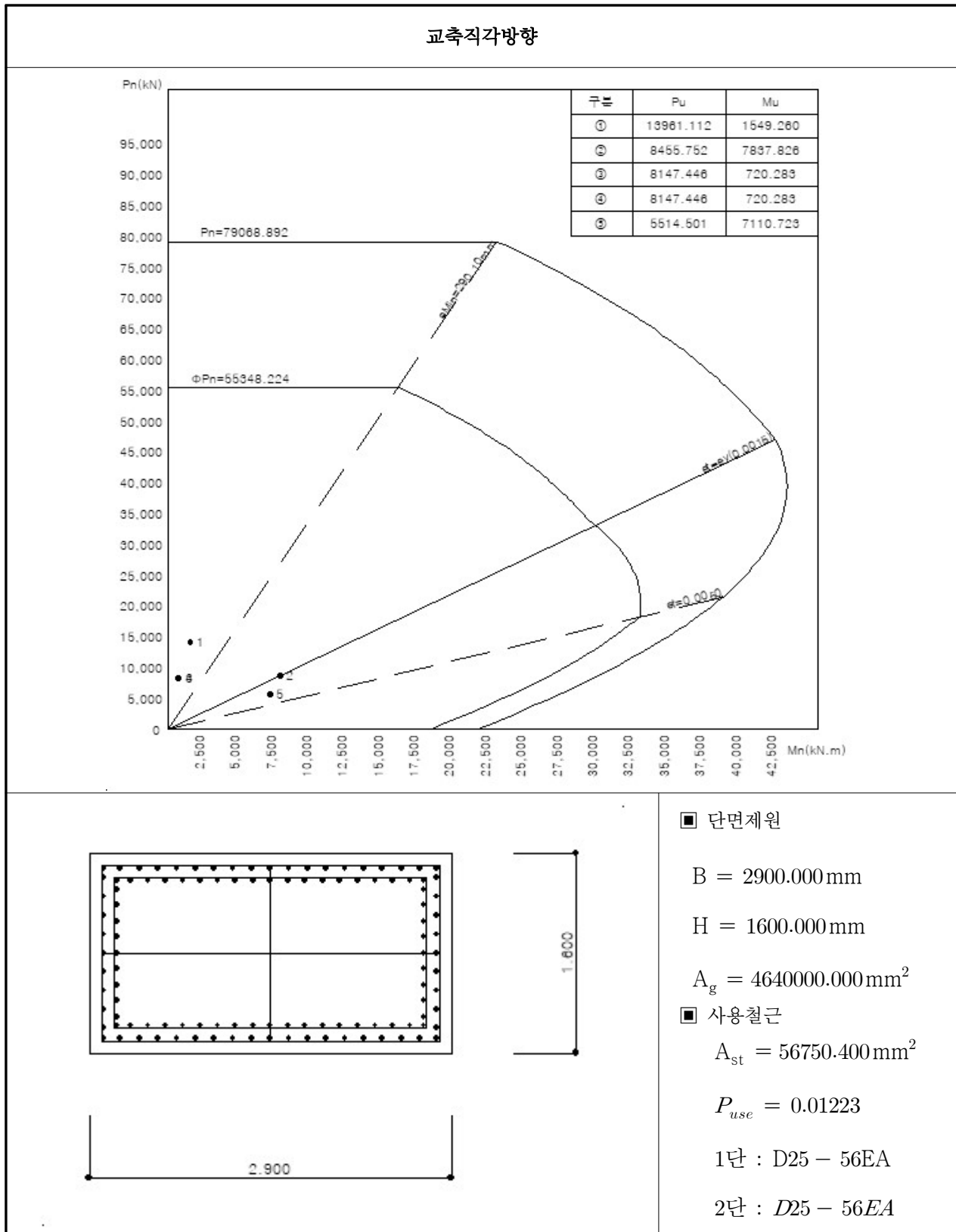
【그림 5.37】 교축직각방향 P-M상관도(P3)(부산)
