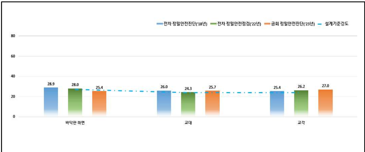
【그림 3.37】 전차 정밀안전진단 및 전차 정밀안전점검 결과 비교(부산)
