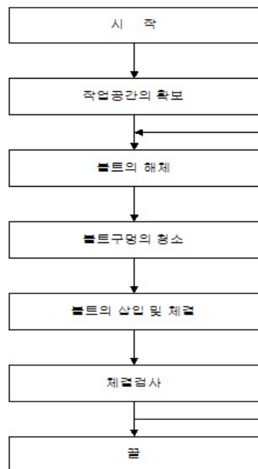
【그림 7.9】 볼트재체결 시공순서도
