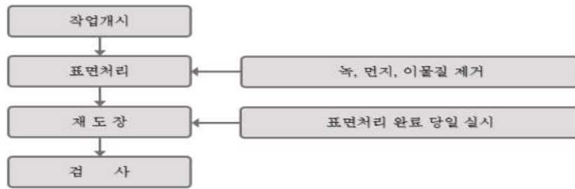
【그림 7.6】 강제 재도장 시공순서도
