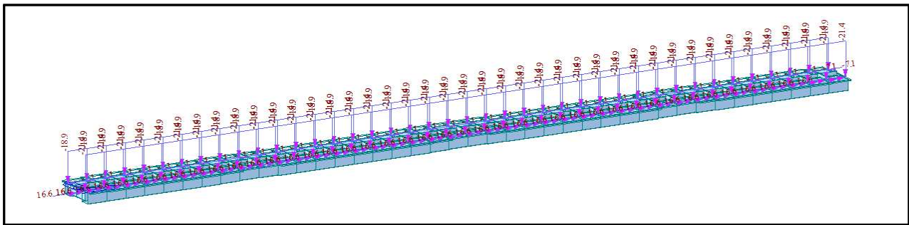
【그림 5.5】 합성 후 고정하중 재하도(부산)
