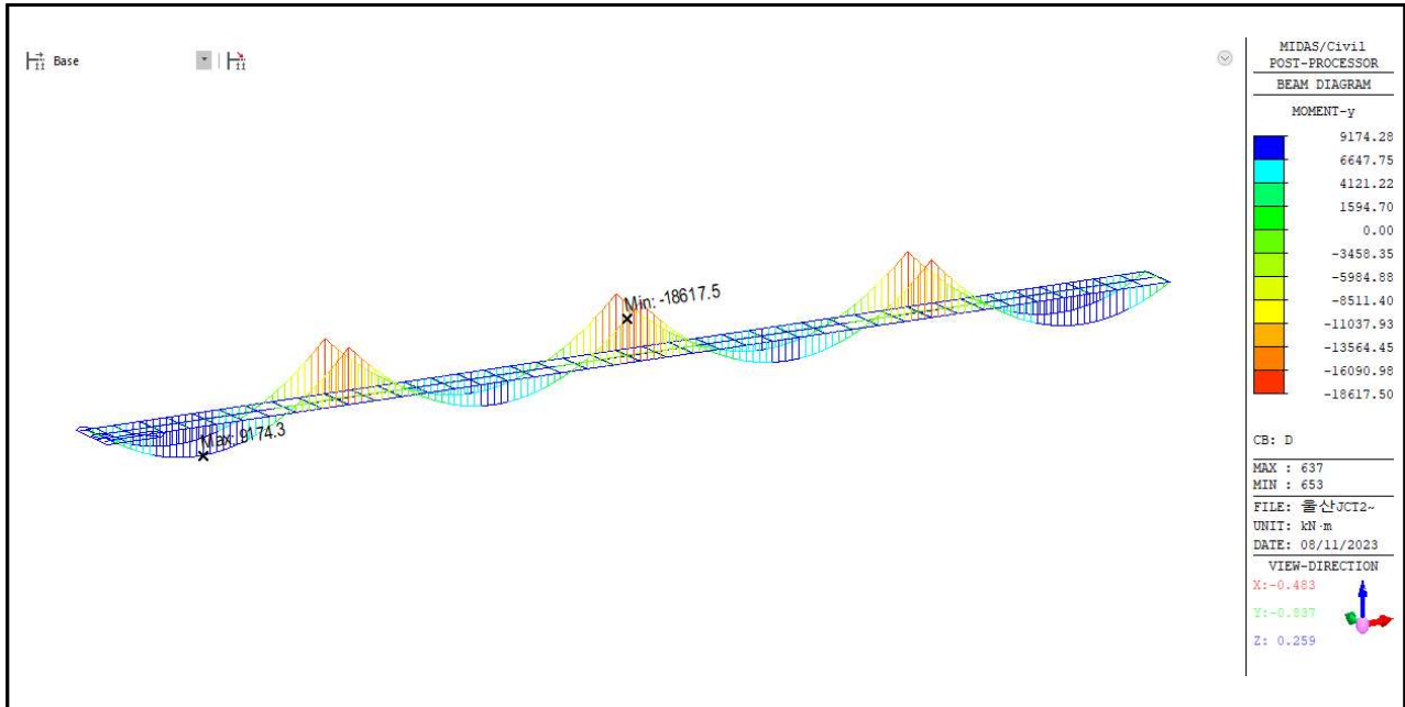
【그림 5.8】 합성전 고정하중에 의한 휨모멘트도(부산)
