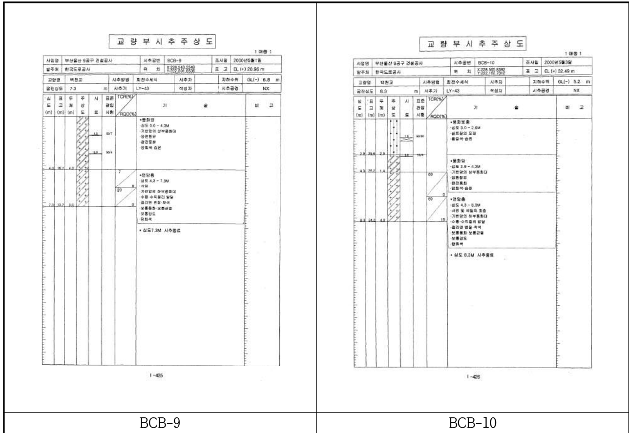
【그림 2.3】 시추조사 주상도(계속)
