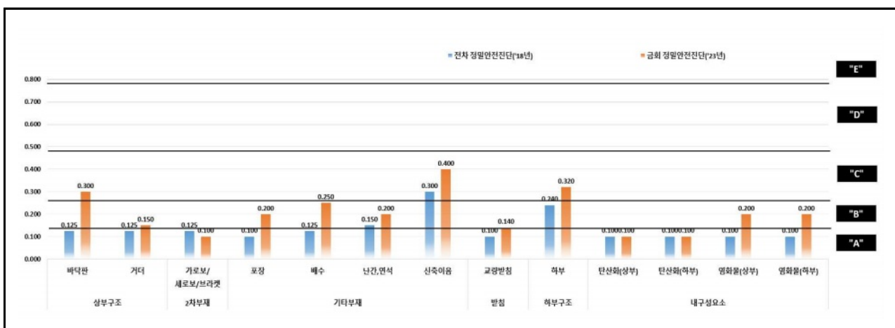
【그림 4.3】 기 진단 결과와의 부재별 상태평가 결과 비교(울산)
