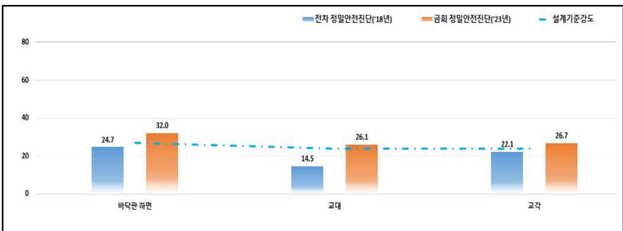
【그림 3.40】 전차 정밀안전진단 결과 비교(부산)
