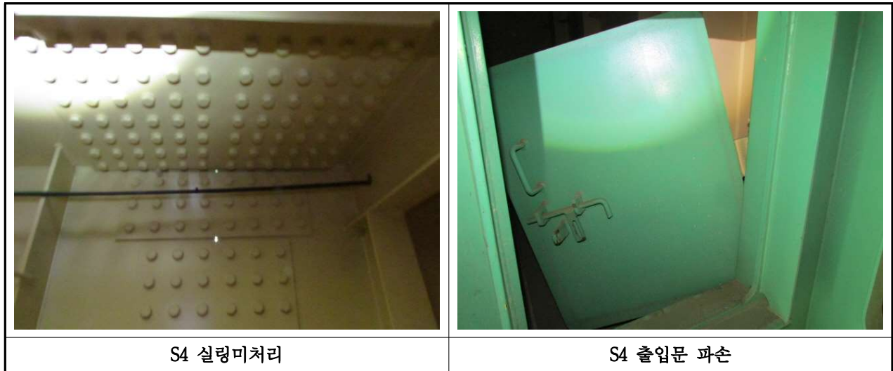
【사진 3.32】강박스 거더 내부 손상현황(울산)
