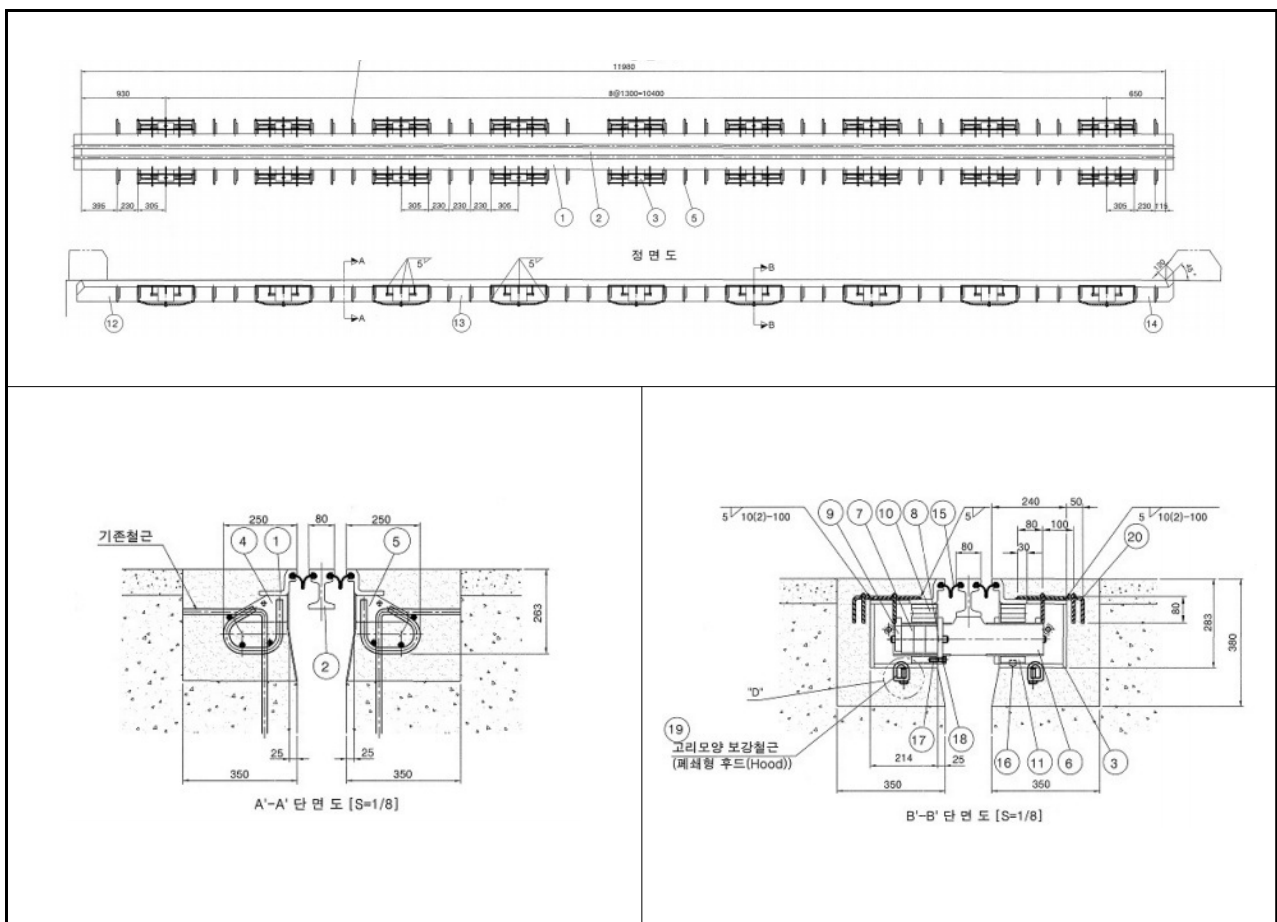
【그림 3.11】 신축이음장치 상세도(부산)
