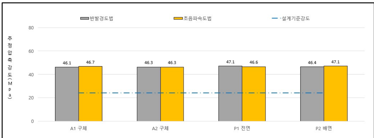
【그림 3.52】하부구조 추정비파괴강도 결과 그래프(울산)
