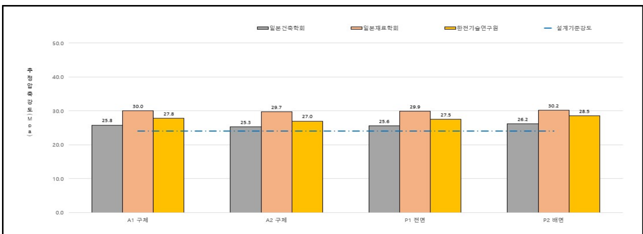
【그림 3.50】 하부구조 초음파 전달속도 시험결과(울산)
