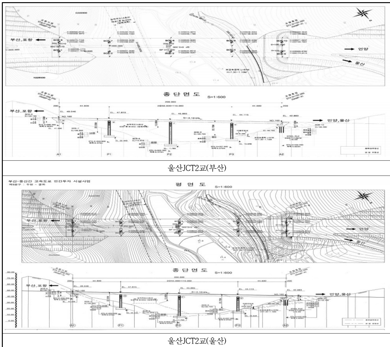
【그림 5.1】 종·평면도
