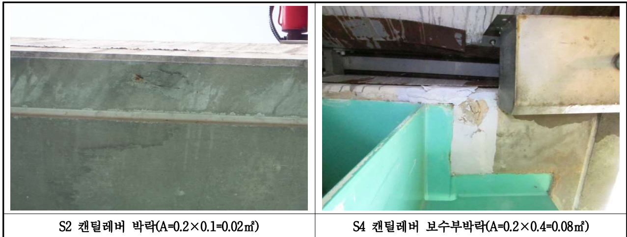
【사진 3.5】 바닥판 손상현황(부산)(계속)
