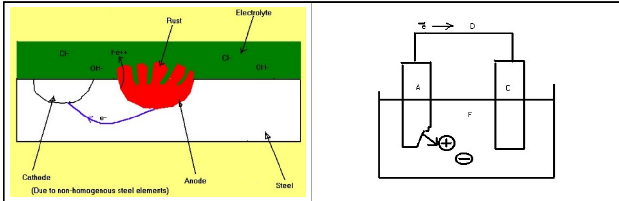
【그림 3.4】 강재의 부식과정 및 원리(부산)
