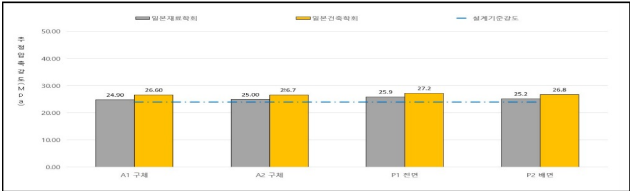
【그림 3.47】 하부구조 반발경도 시험결과(울산)
