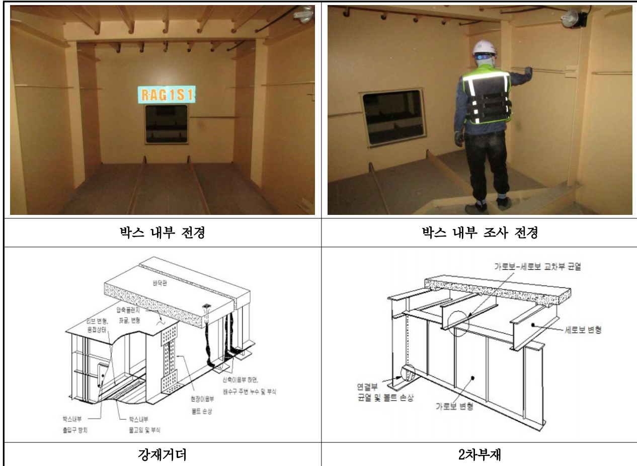
【사진 3.7】강박스 거더 전경 및 일반적인 손상(부산)
