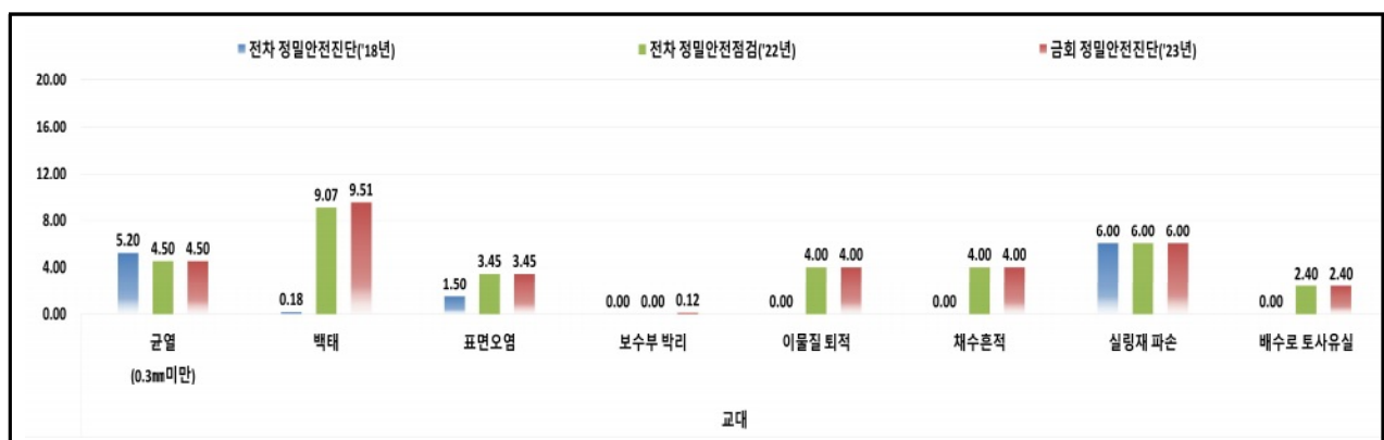
【그림 3.23】 교대 기 점검 결과와의 비교(울산)
