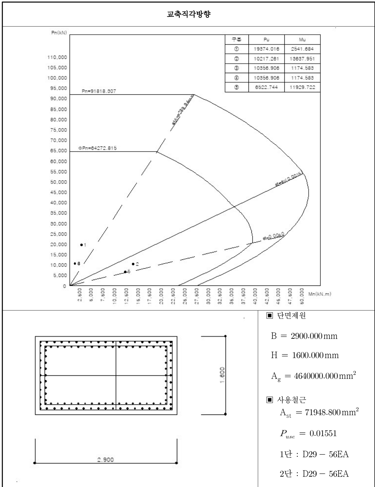
【그림 5.42】 교축직각방향 P-M상관도(P2)(울산)
