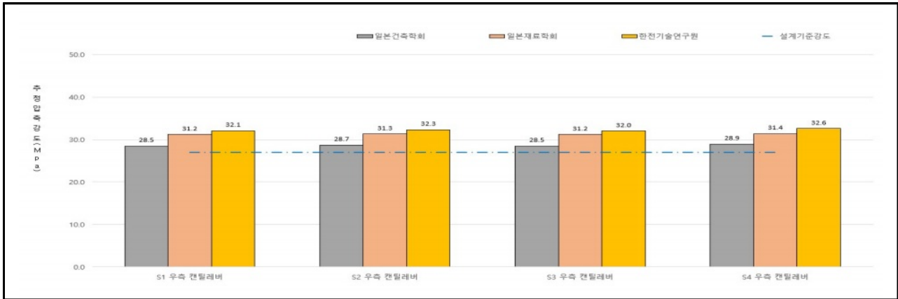
【그림 3.38】 상부구조 초음파 전달속도 시험결과(부산)
