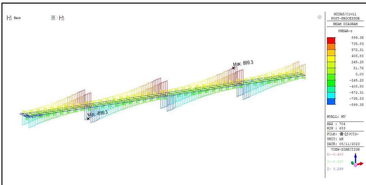
【그림 5.13】 활하중에 의한 전단력도(부산)
