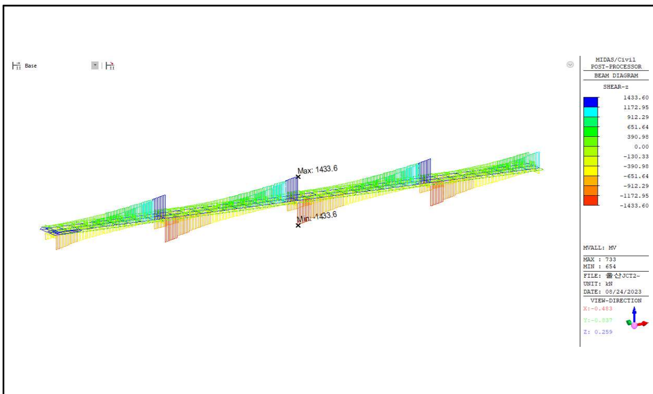
【그림 5.27】 활하중에 의한 전단력도(울산)
