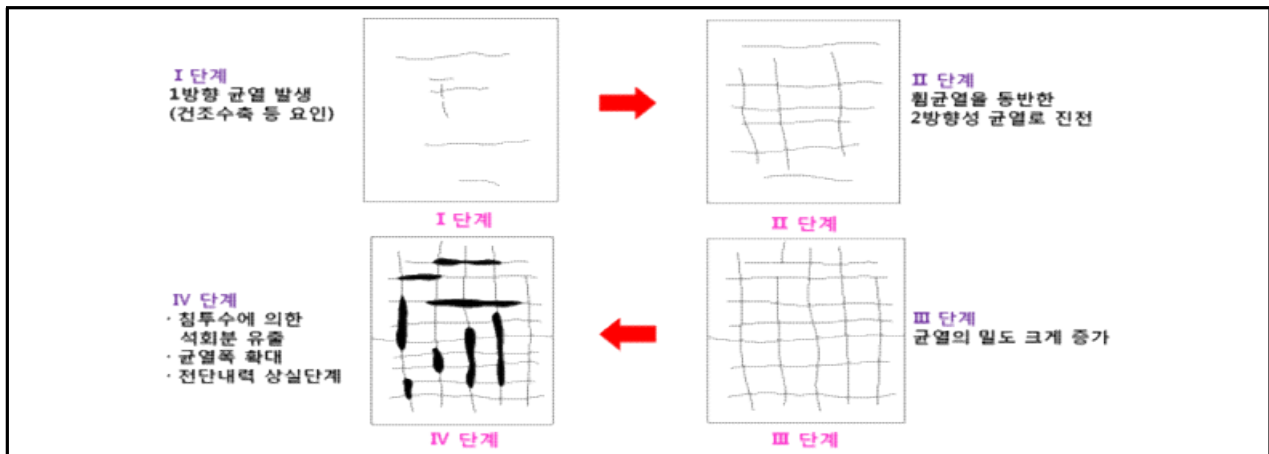
【그림 3.18】 콘크리트 바닥판의 균열진전 개요도(울산)
