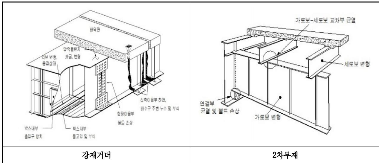
【그림 3.19】 강박스 거더의 일반적인 손상(울산)
