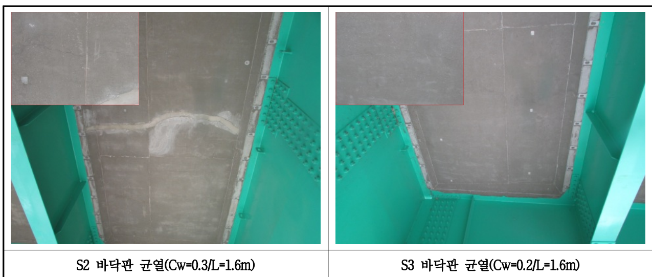
【사진 3.5】 바닥판 손상현황(부산)
